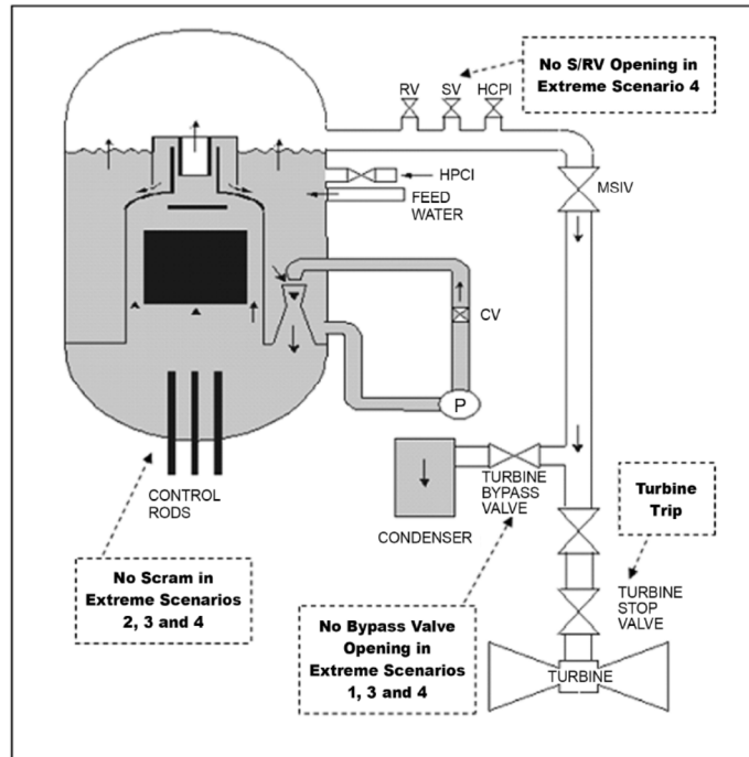
図2 BWR タービントリップベンチマーク問題 Exercise 3 シナリオ 1~4 (文献[8]図 2-1)
