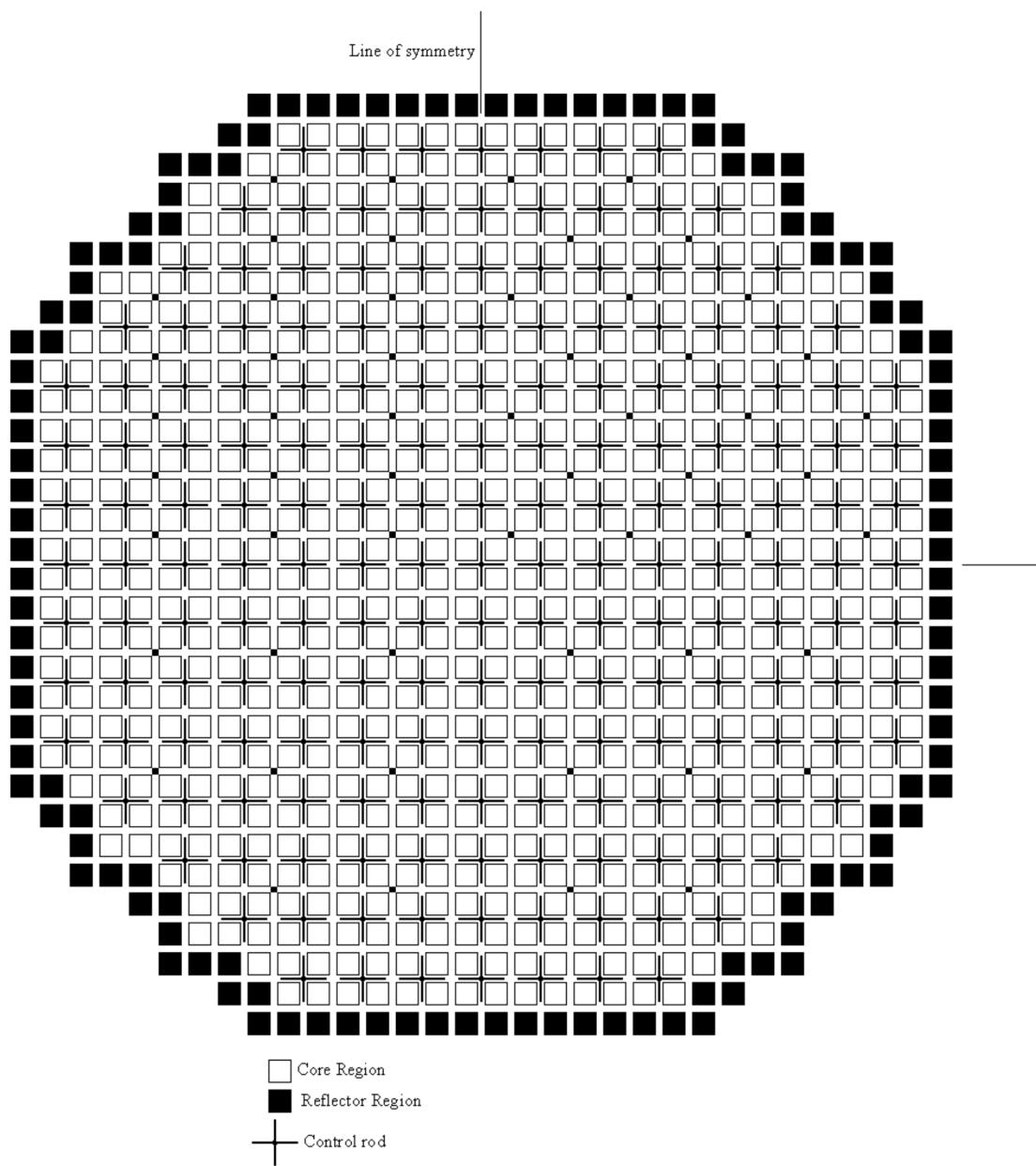
図1 PB-2 炉心における燃料集合体及び制御棒位置 (文献[7] 図 2-1)
