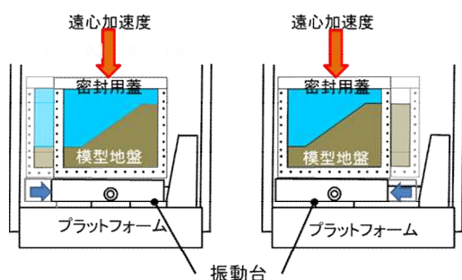
図1 遠心場における振動台による動的载荷のイメージ
