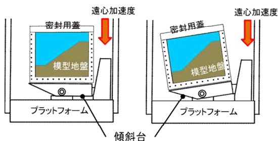
図4 遠心場における傾斜台による静的载荷の概念図
