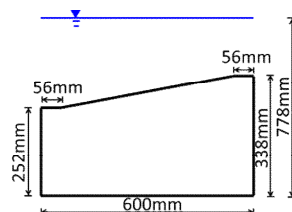
図3 模型地盤(傾斜角10°)
