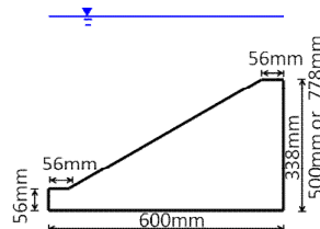
図2 模型地盤(傾斜角30°)
