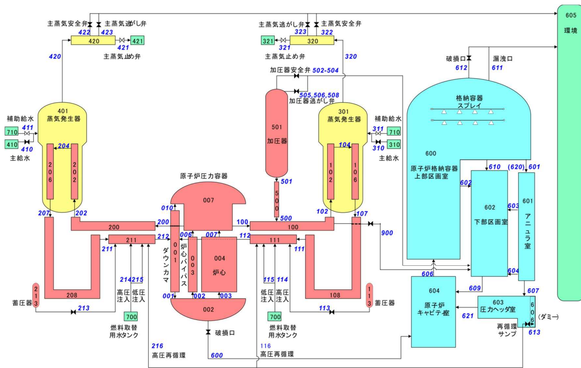
図 1 PWR プラントのノード分割及びフローパスの関係図 4) (イメージ)
