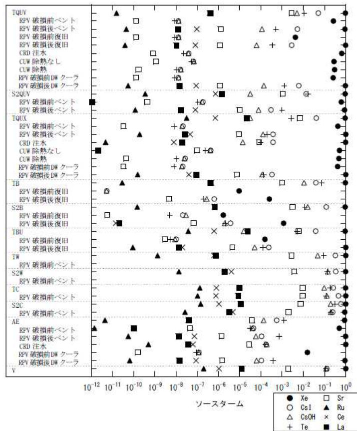
図3 代表的な事故シーケンスの放出量 5) (イメージ)
