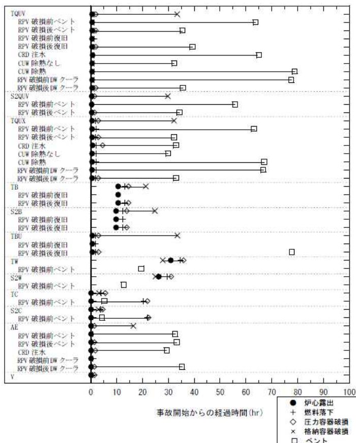
図 2 代表的な事故シーケンスの事象進展タイミング 5) (イメージ)
