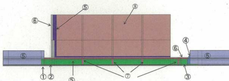
低圧用電気ペネトレーション解析モデル
