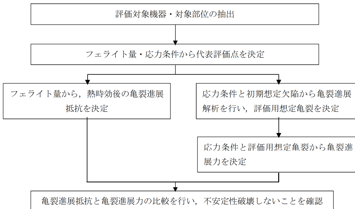
図1 熱時効評価フロー
