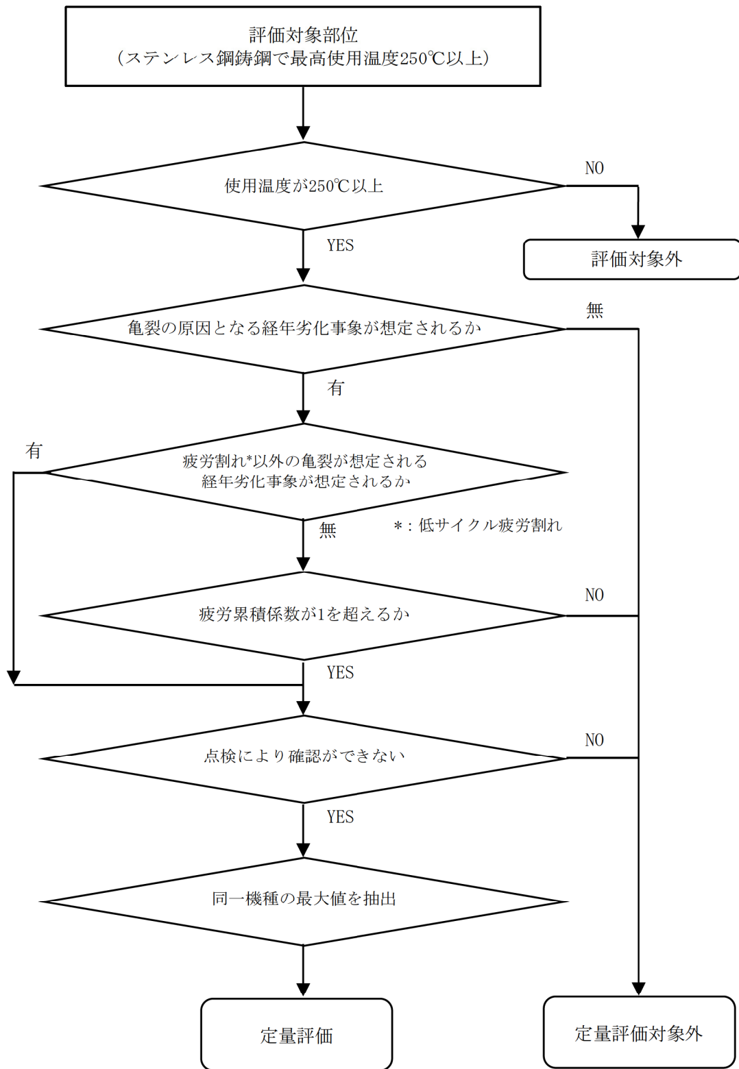
図2 熱時効スクリーニングフロー
