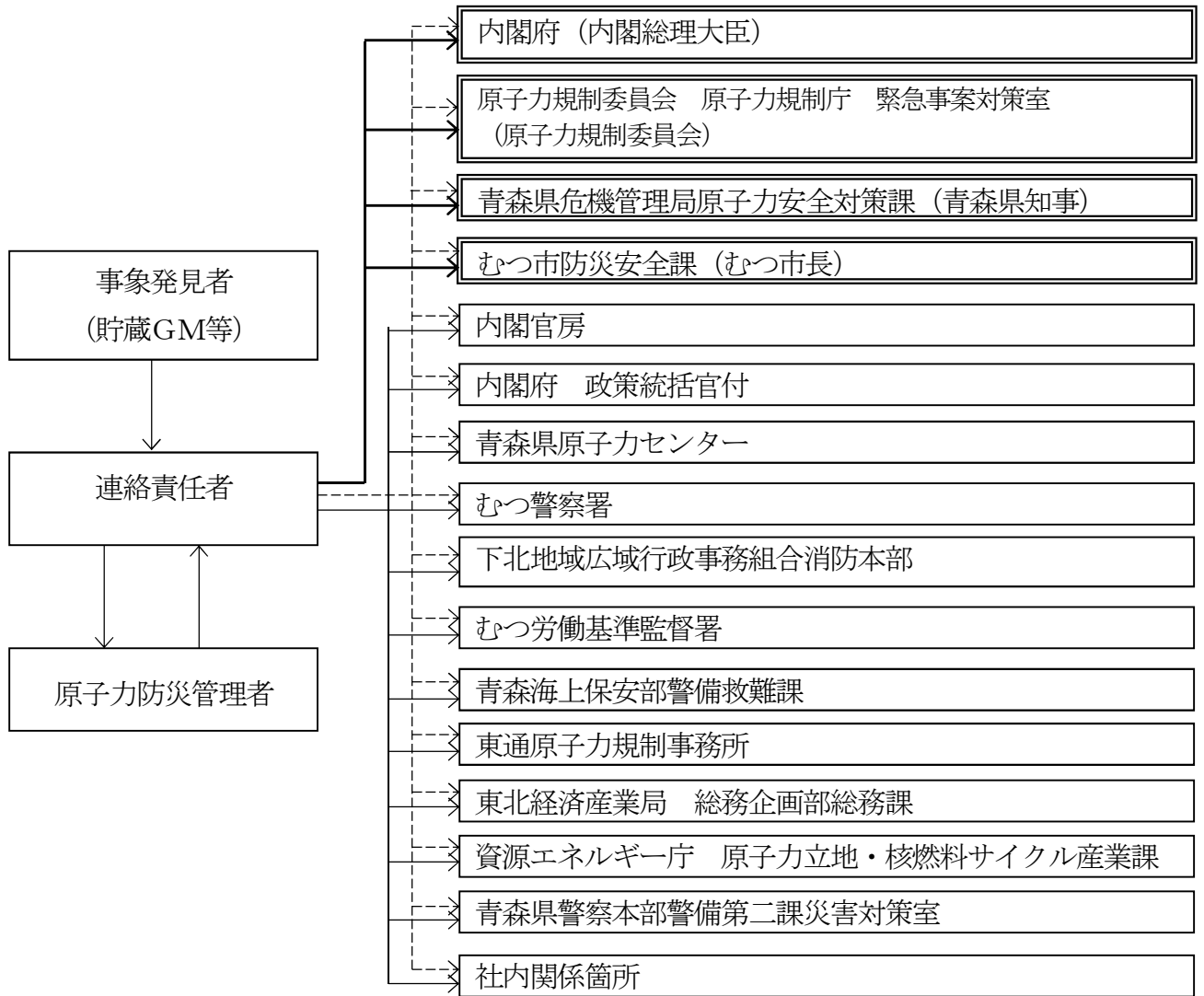
別図 2-3 原子力災害対策特別措置法第 10 条第 1 項に基づく通報経路 備蓄センター内での事象発生時の通報経路
