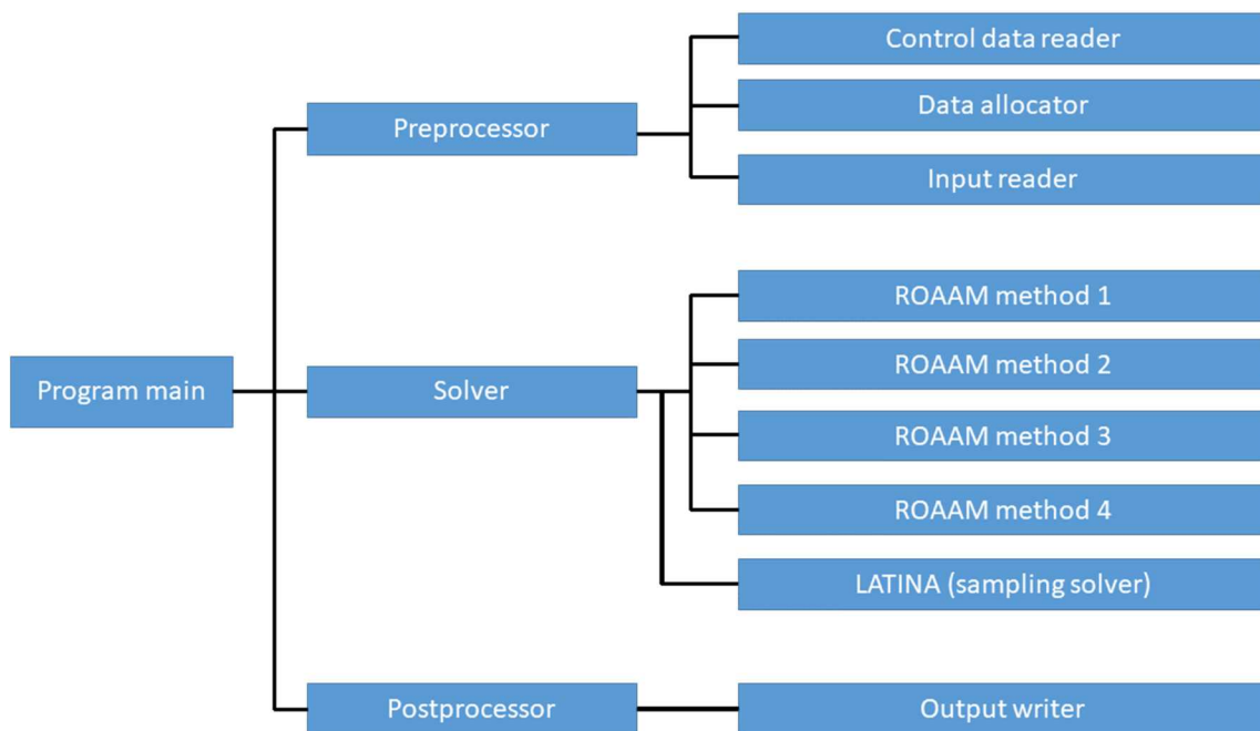
図 1 プログラム構造の例
