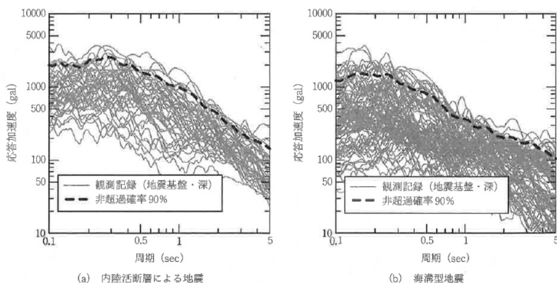
図4-2 【参考】鉄道構造物等設計標準・同解説 1) による応答スペクトルの分析結果： L2地震動における観測記録の応答スペクトル（地震規模、震源距離、地盤条件の補正有）
