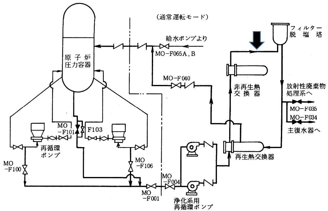
図 東海第二発電所 原子炉冷却材浄化系概略図 (サンプリング点は➡部)
