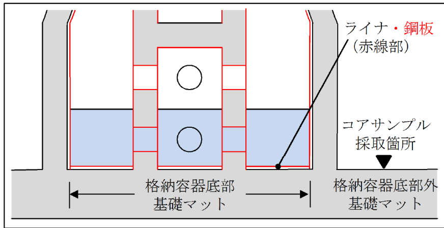
図 4. 1. 1-1 格納容器底部基礎マット概要図
