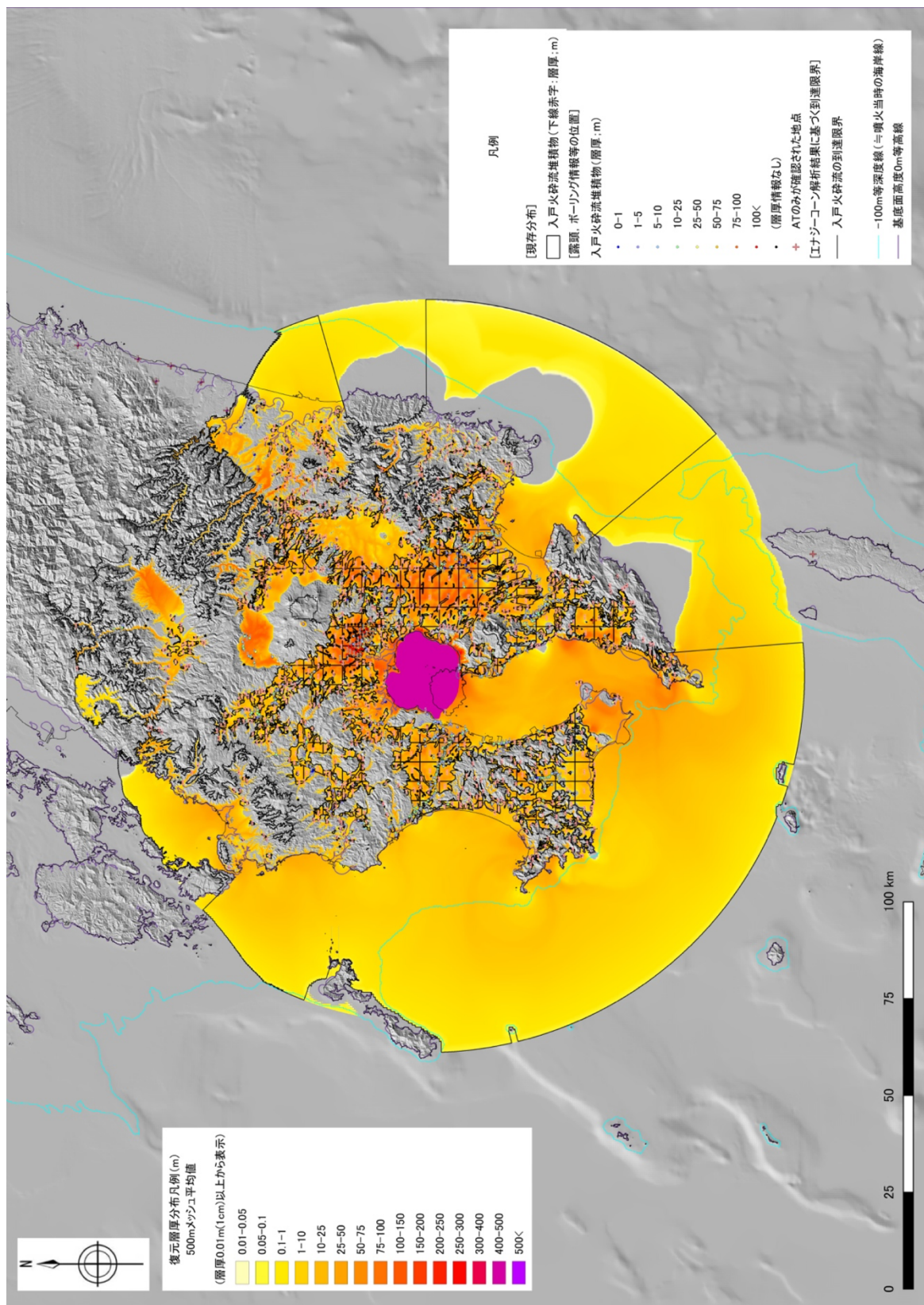
図 1.5-23b. 復元層厚分布 (500m メッシュ平均値)
