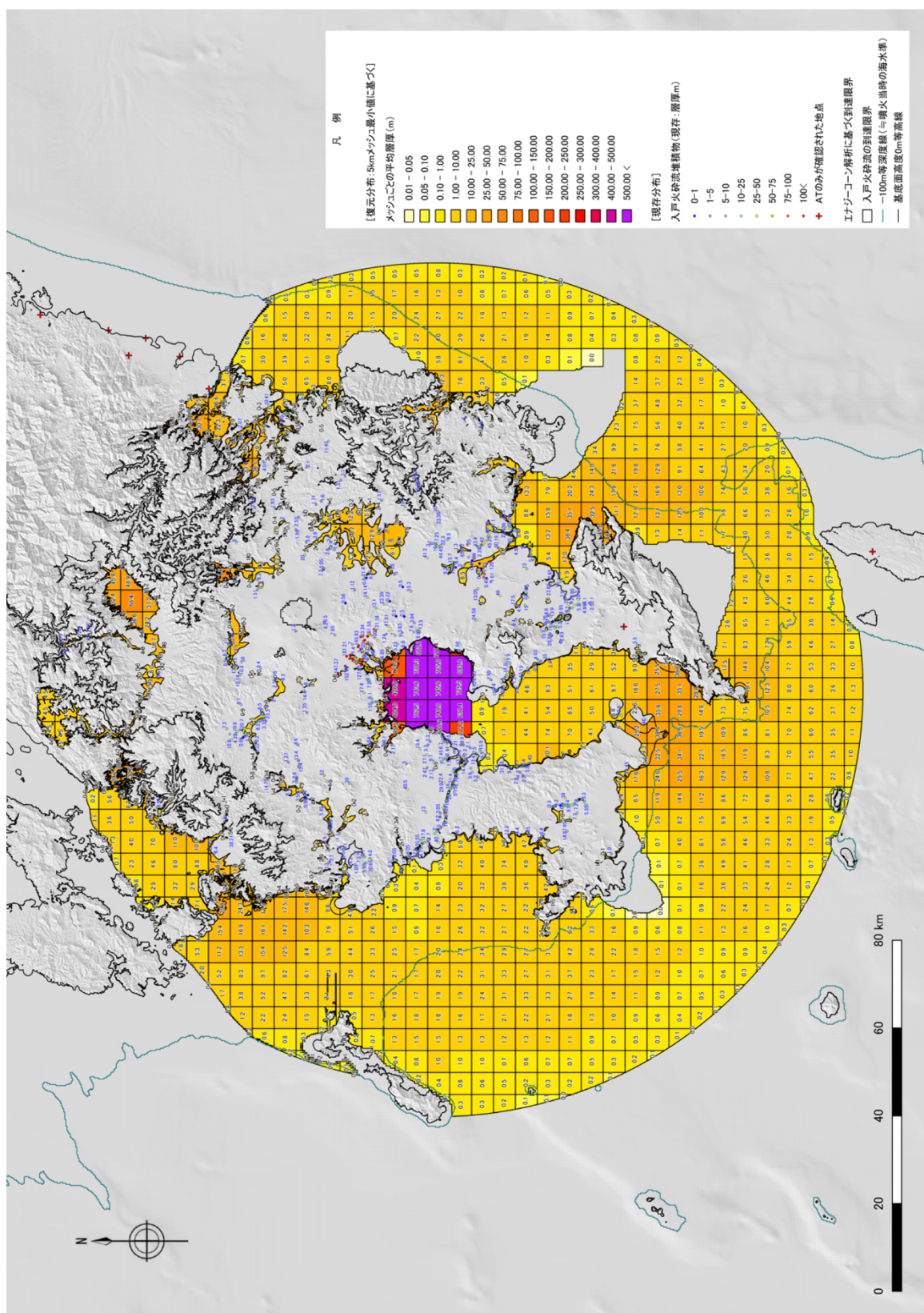
図 1.5-24c. メッシュごとの平均層厚 (メッシュサイズ: 5km 最小値)
