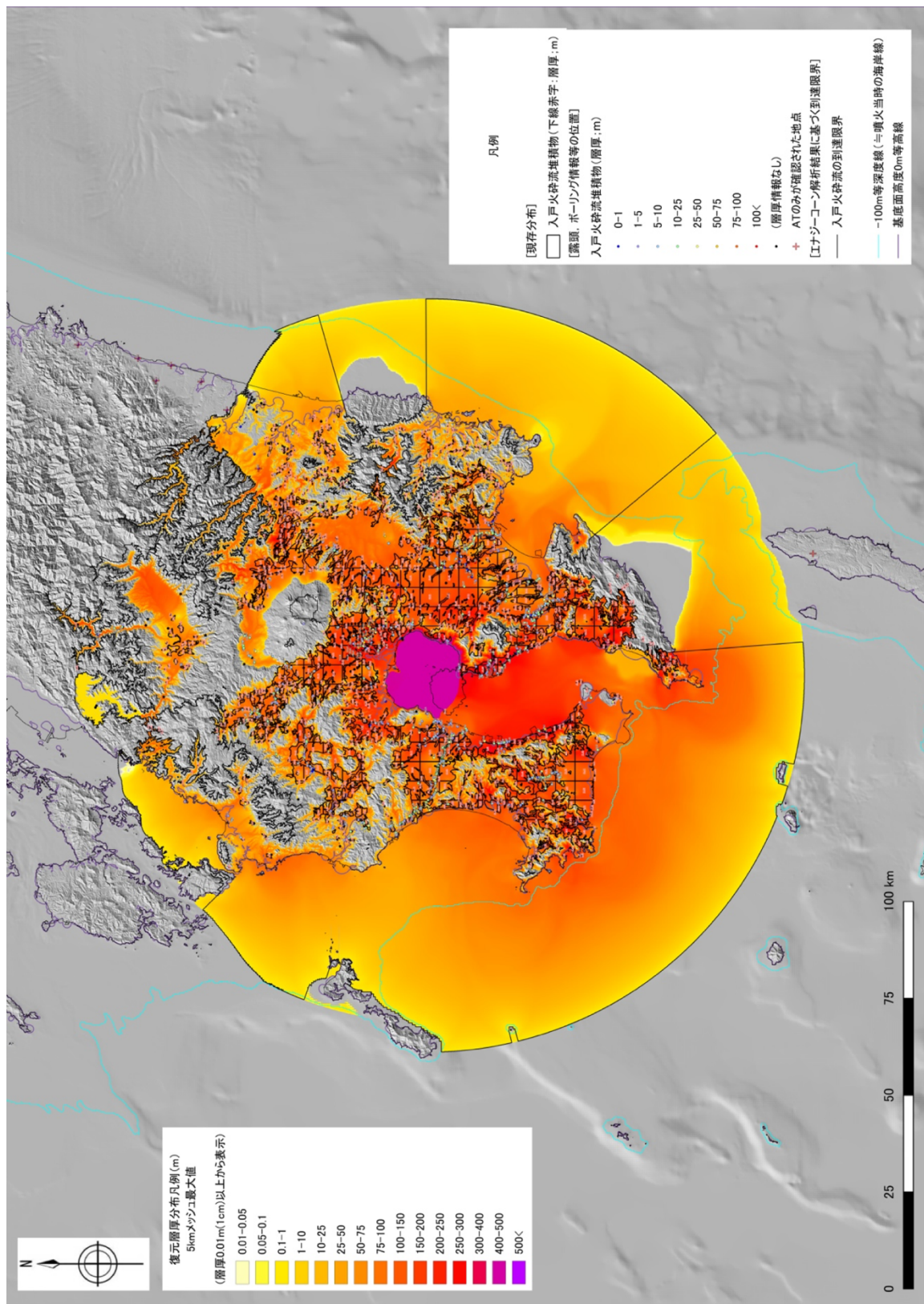
図 1.5-23g. 復元層厚分布 (5km メッシュ最大値)
