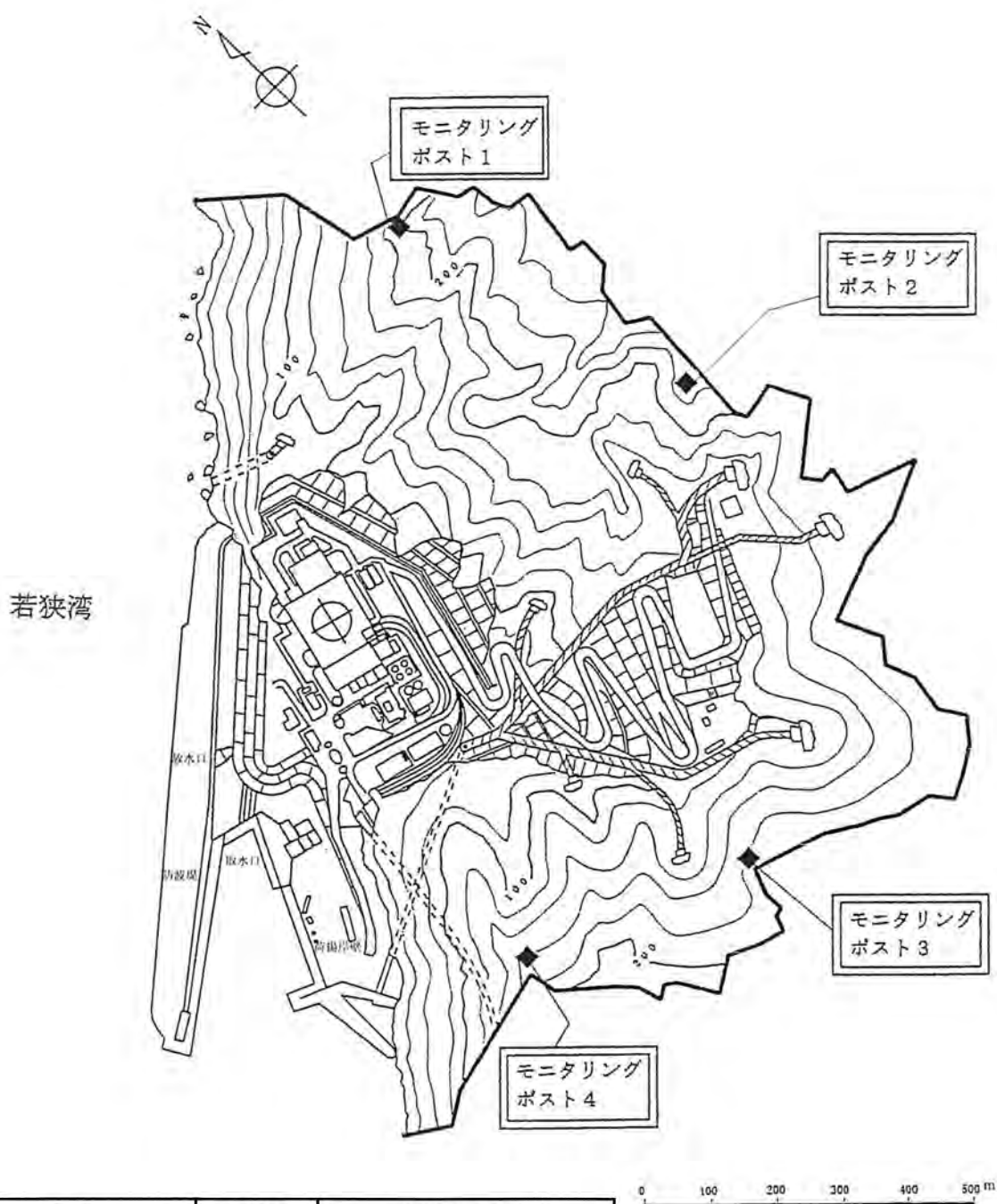
別図2-3-10 もんじゅ敷地境界付近の放射線測定設備
