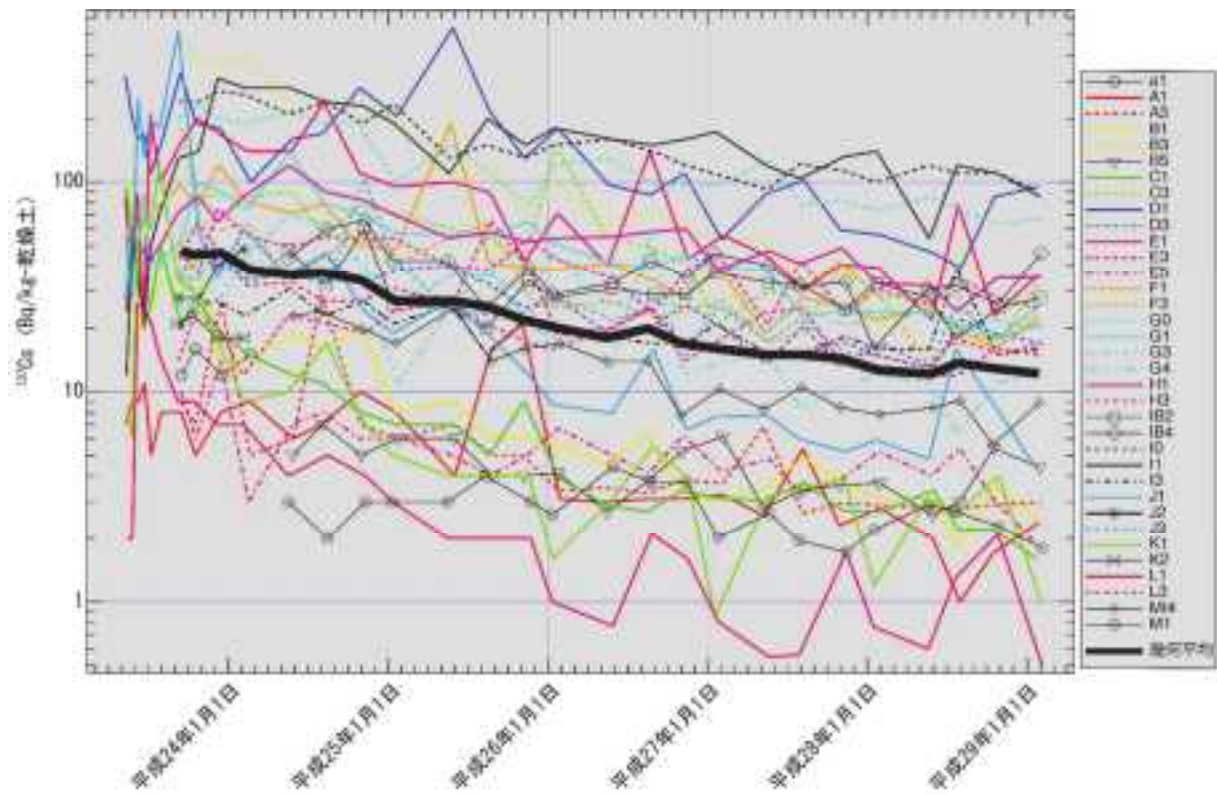
図 II-3-14 各測点における ^{137}\text{Cs} 濃度の時系列変化
