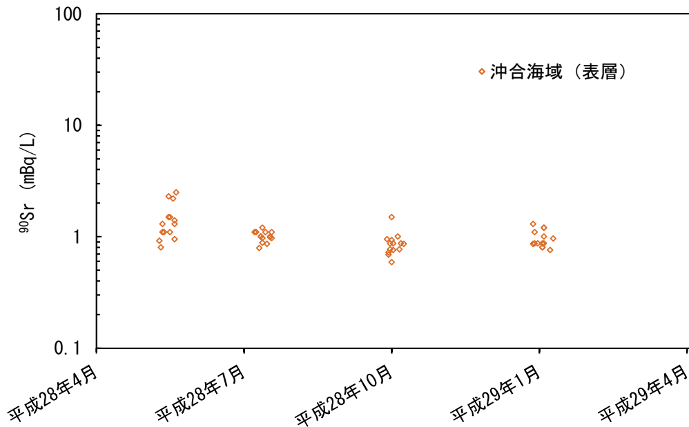
図Ⅱ-3-7 沖合海域における ^{90}\text{Sr} 濃度の時系列変化
