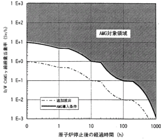
ドライウエル領域のγ線線量率
