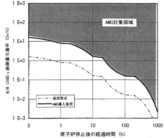
サプレッションチェンバ領域のγ線線量率
