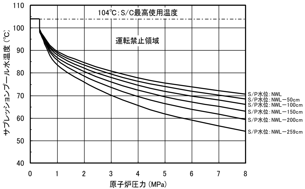
サプレッションプール 熱容量制限図
