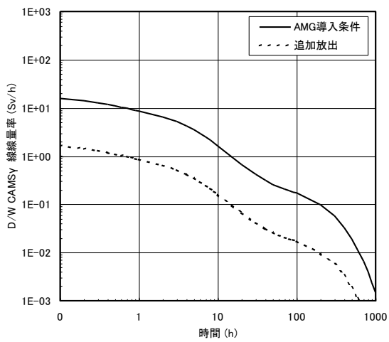
ドライウエル領域のγ線線量率
