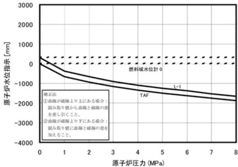
原子炉圧力変化に対する燃料域水位計補正曲線
