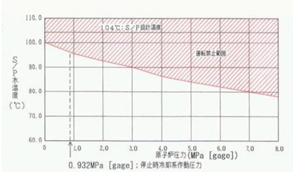
サプレッションプール 熱容量制限図
