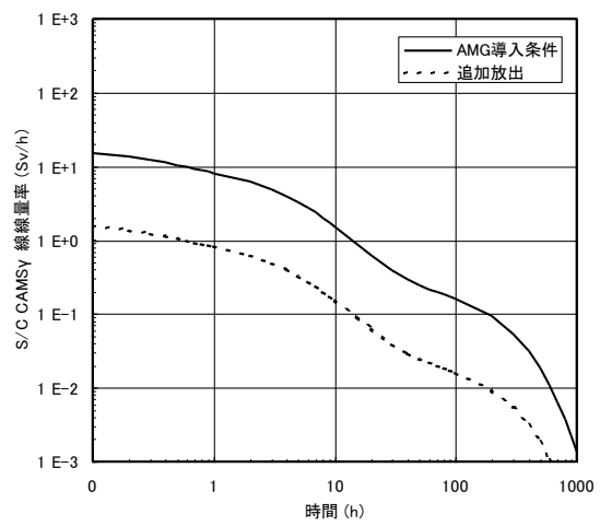
サプレッションチェンバ領域のγ線線量率
