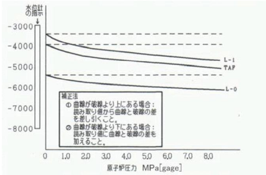
原子炉圧力変化に対する燃料域水位計補正曲線
