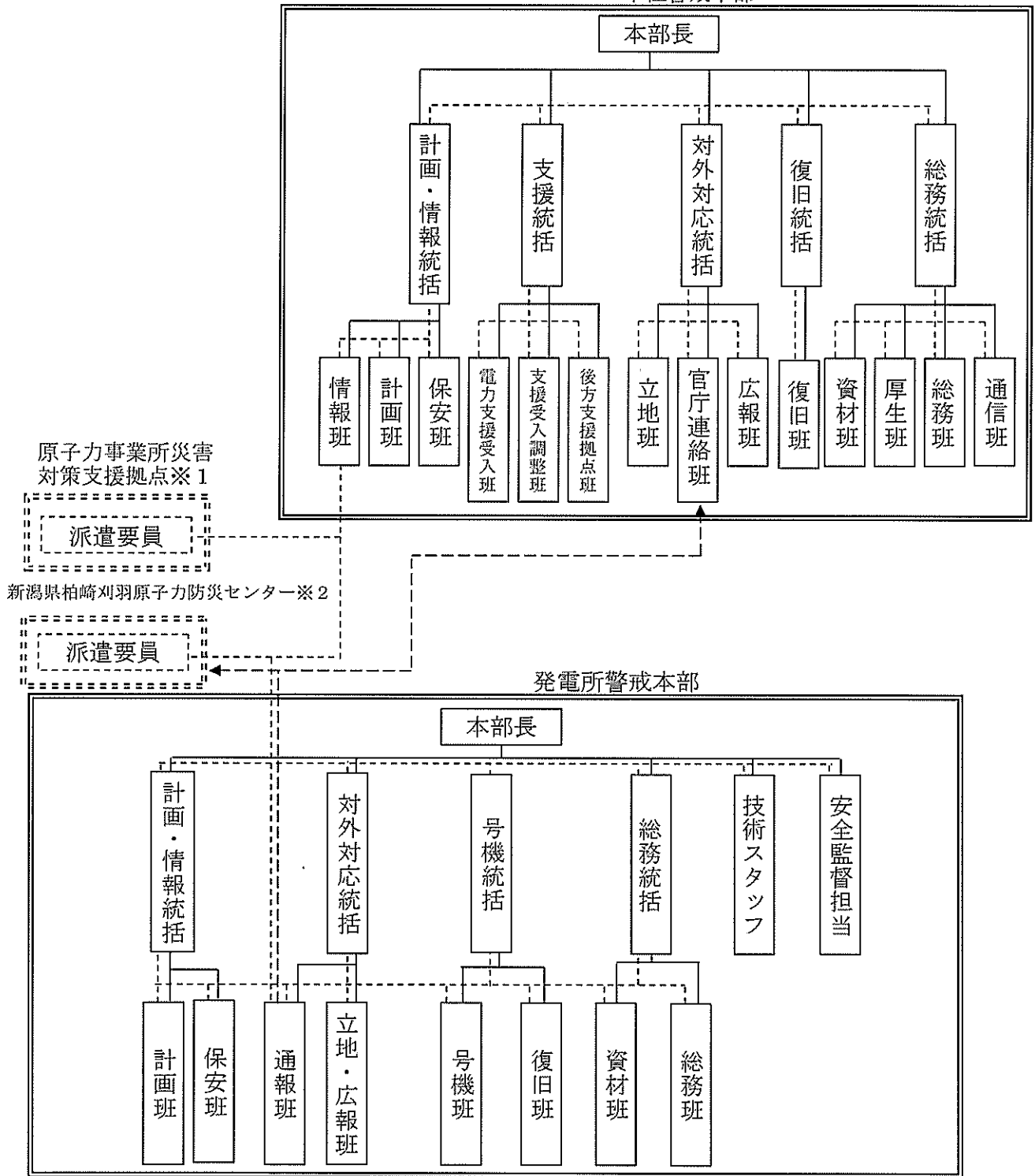
別図2-6 原子力警戒態勢発令後の社内の伝達経路 本社警戒本部
