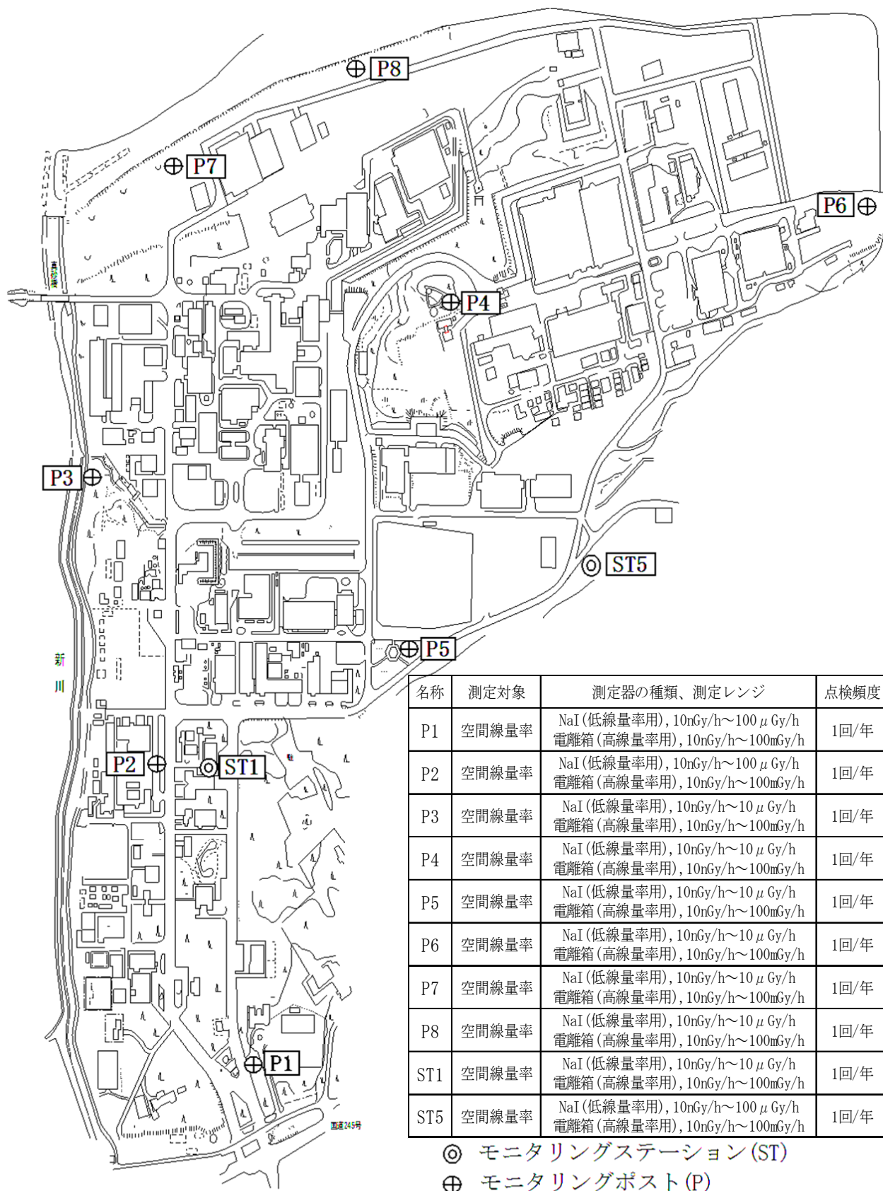
別図－４ サイクル研究所敷地周辺の放射線測定設備
