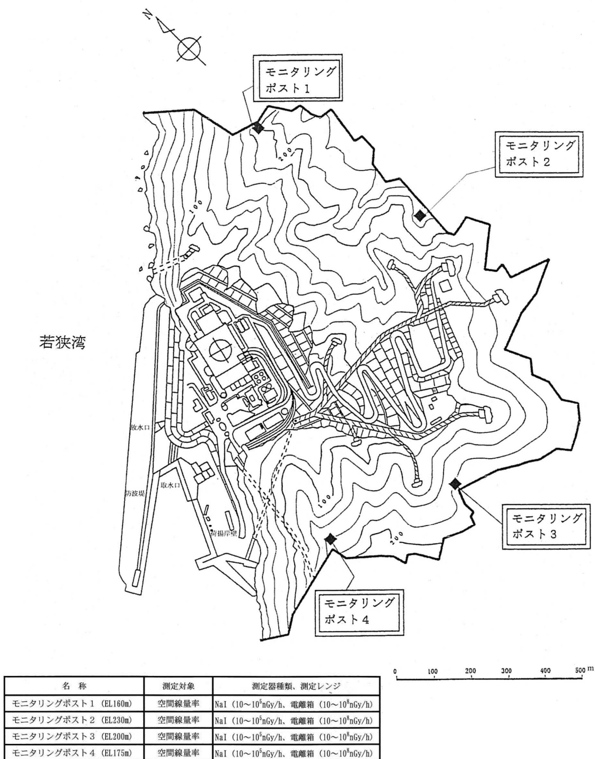
別図 2-3-10 もんじゅ敷地境界付近の放射線測定設備
