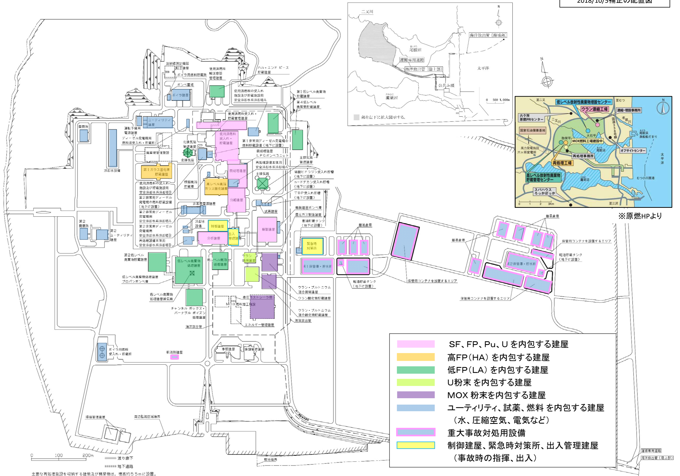
第4図 再処理施設一般配置図（その3）
