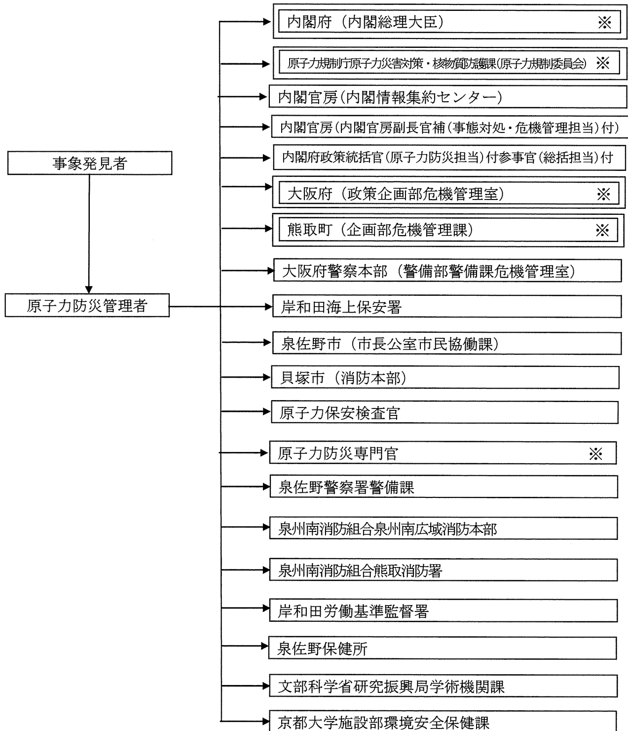
別図第3—1 原災法第10条第1項に基づく通報経路 実験所内での事象発生時
