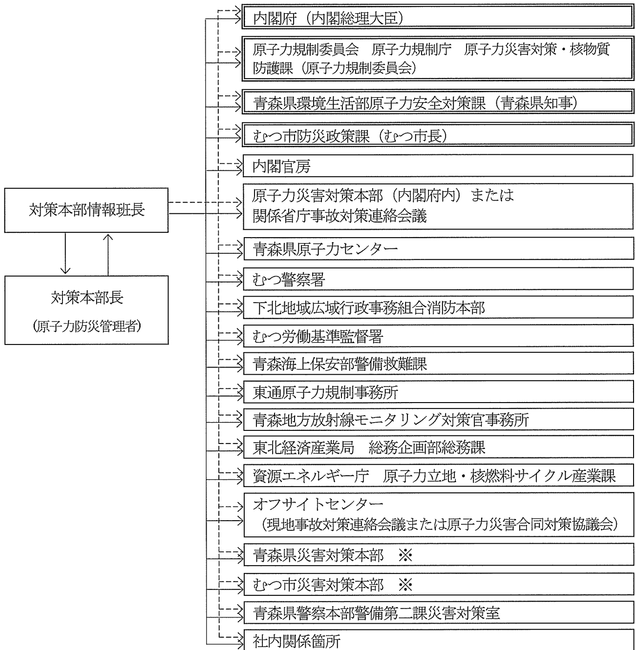
別図 2-4 原子力災害対策特別措置法第 10 条第 1 項の通報後の連絡経路 備蓄センター内での事象発生時の連絡経路
