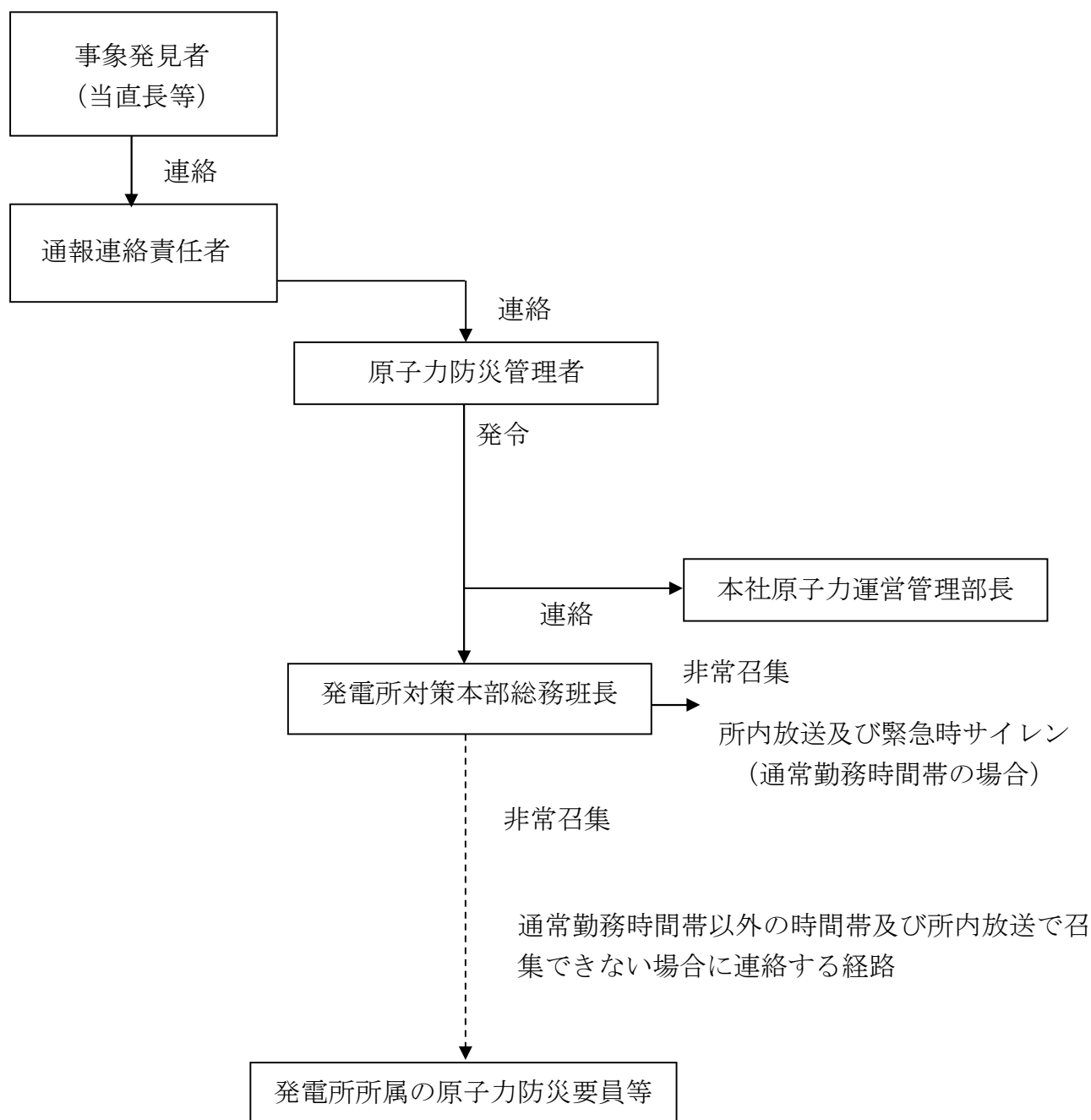
別図 2－8 発電所における原子力警戒態勢発令及び緊急時態勢発令と 発電所所属の原子力防災要員等の非常召集連絡経路
