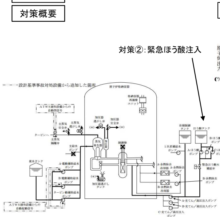
対策①: ATWS緩和設備の作動
