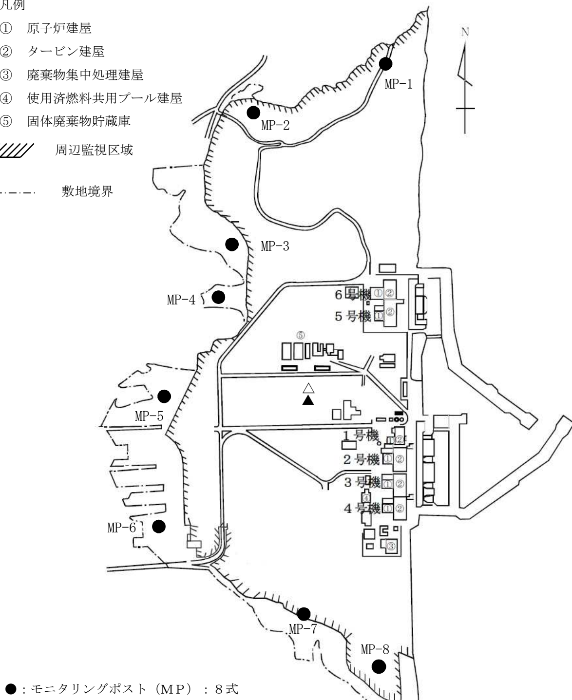
別図 2 - 1 0 発電所敷地周辺の放射線測定設備等
