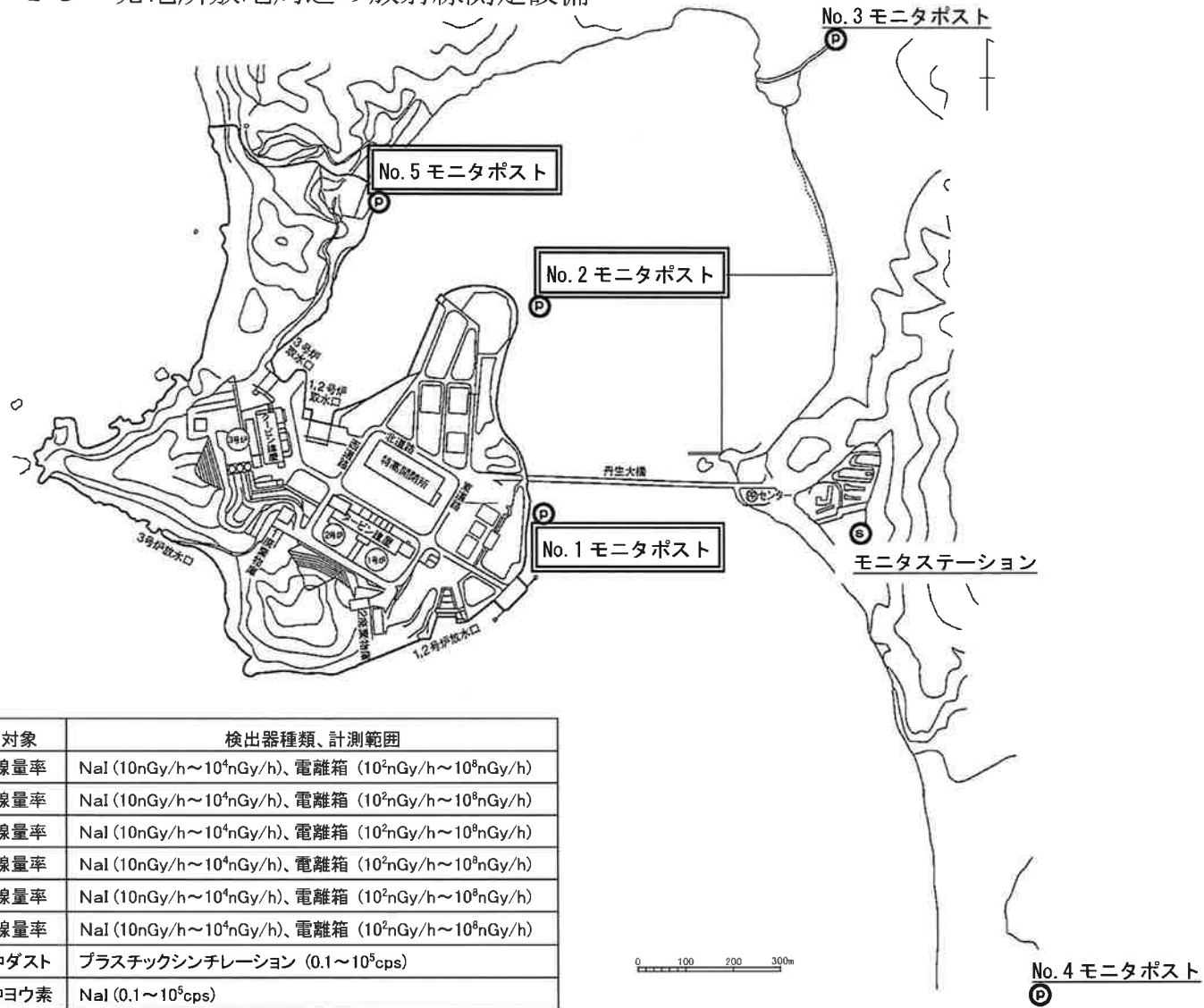
別図 2－3－1 3 発電所敷地周辺の放射線測定設備
