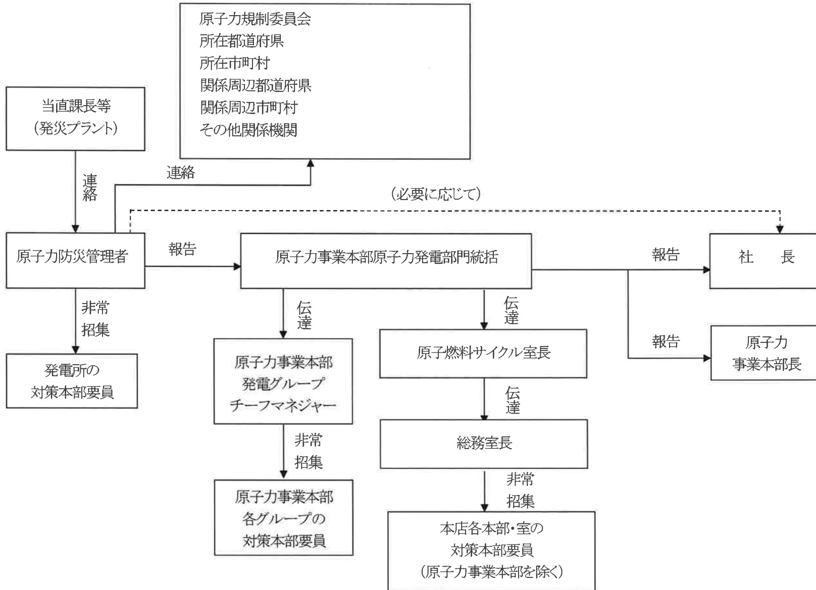
別図2-2-7 警戒体制および原子力防災体制発令時の連絡経路
