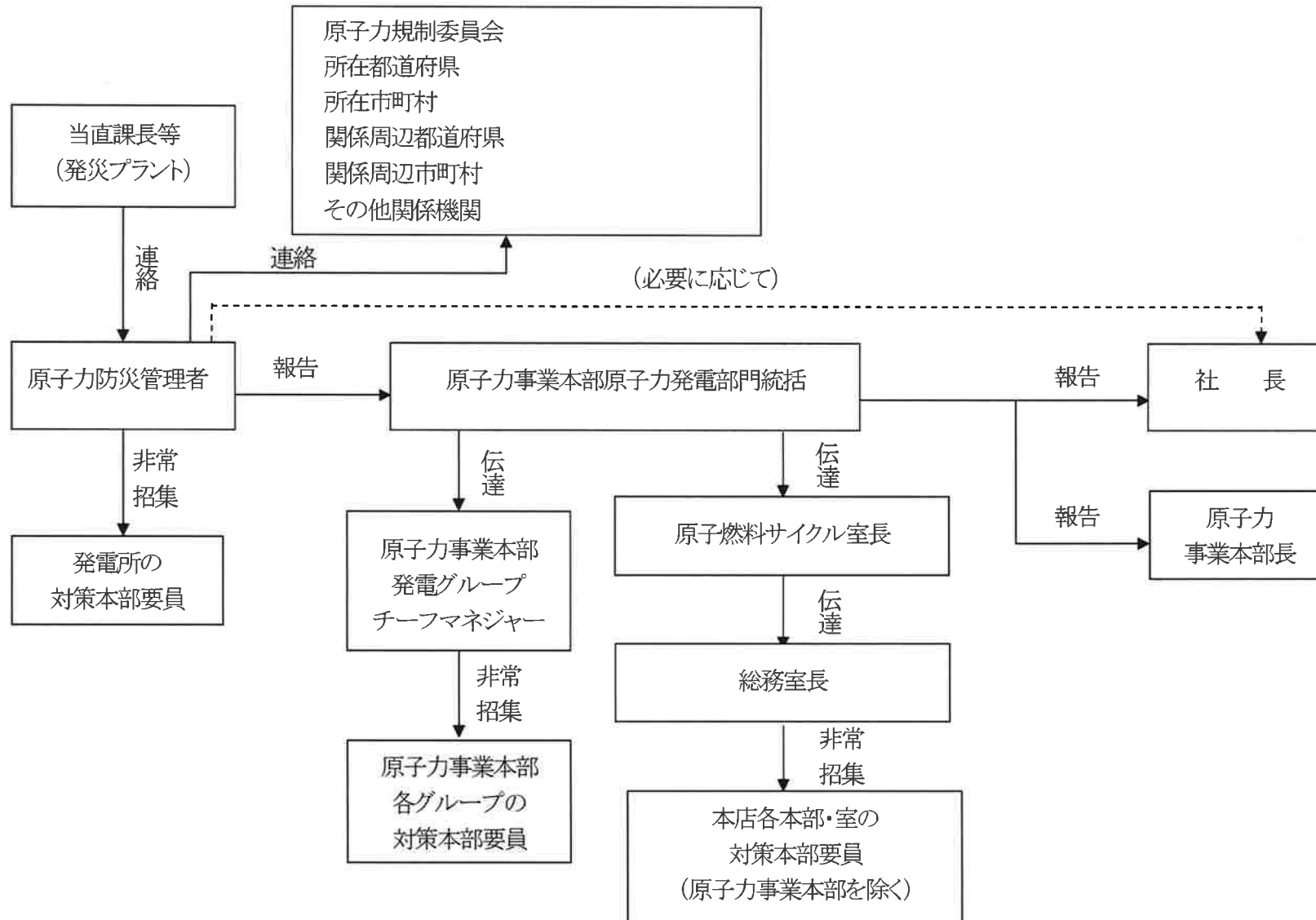
別図2-2-7 警戒体制および原子力防災体制発令時の連絡経路
