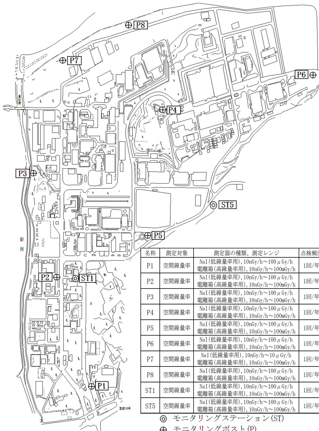
別図ー 4 サイクル研究所敷地周辺の放射線測定設備
