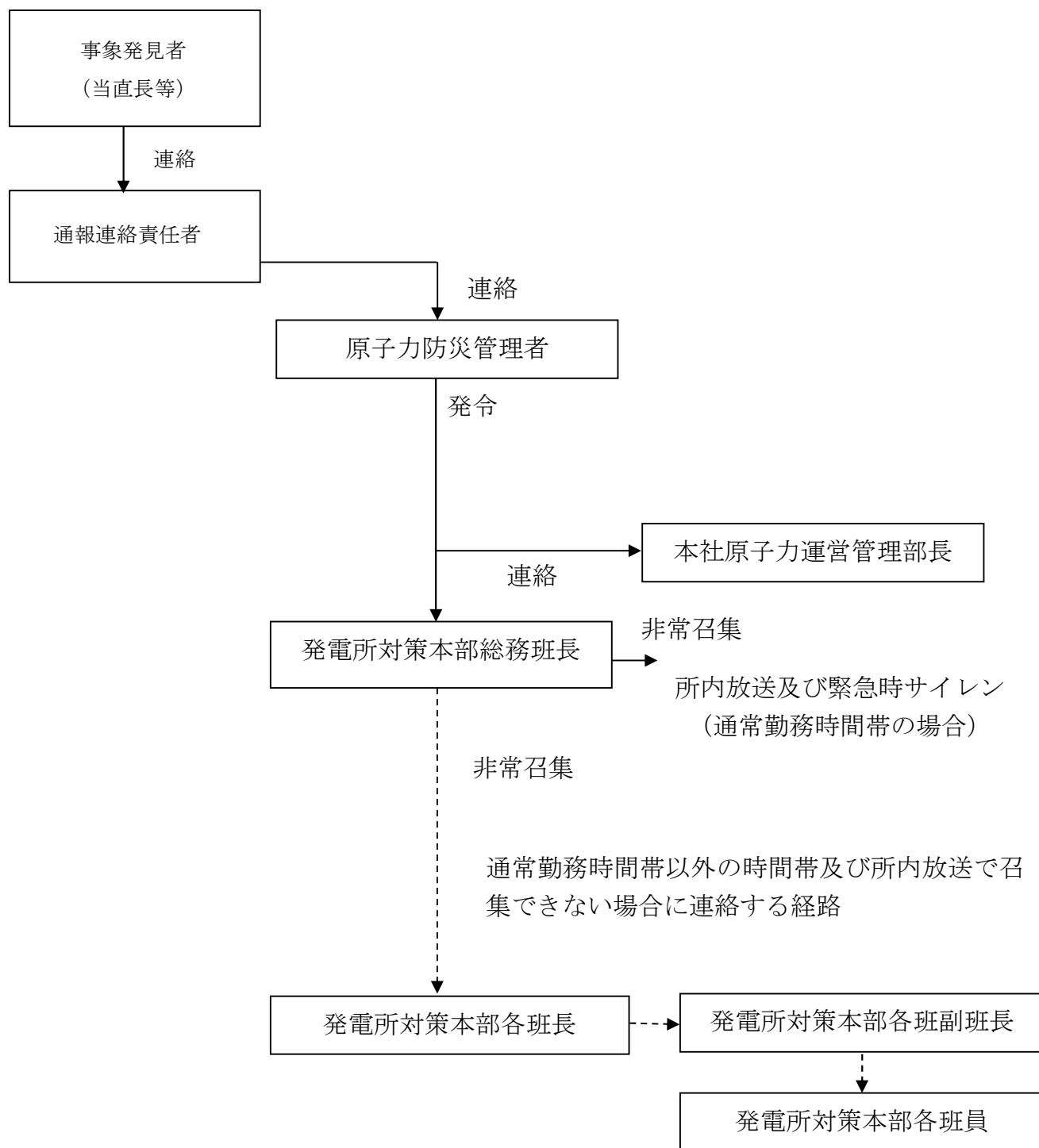
別図 2－8 発電所における原子力警戒態勢発令及び緊急時態勢発令と 緊急時対策要員の非常召集連絡経路
