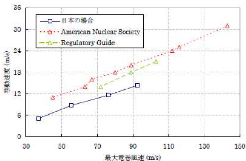
解説図 3.6 竜巻の移動速度と最大風速の関係 (参 3)
