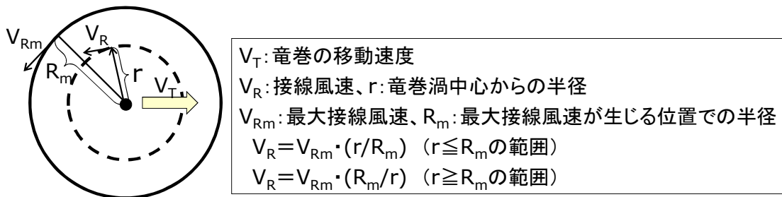
解説図 3.5 ランキン渦モデルの概要
