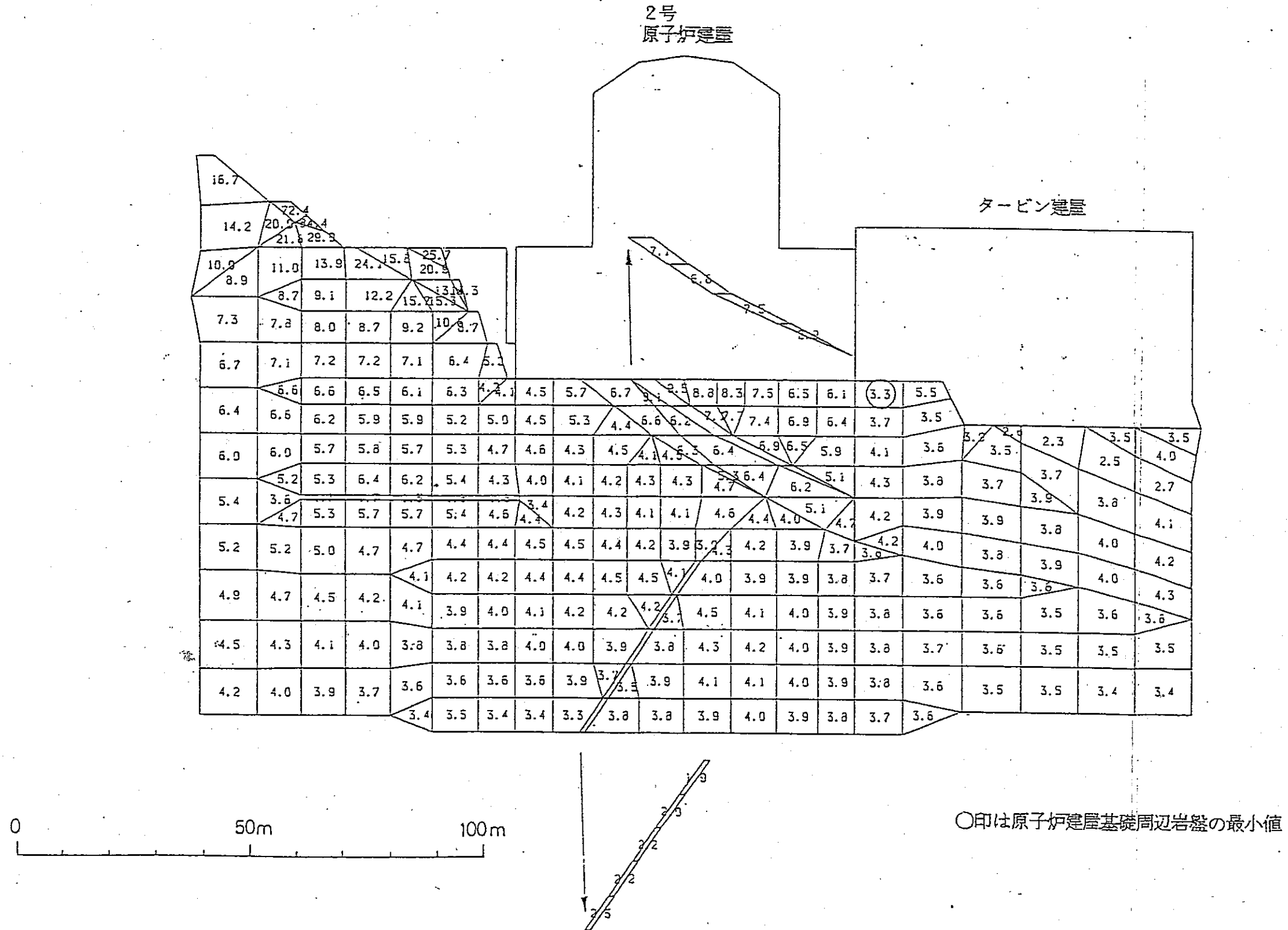
第3.148図 地震時局所安全係数図 (主要部分)
