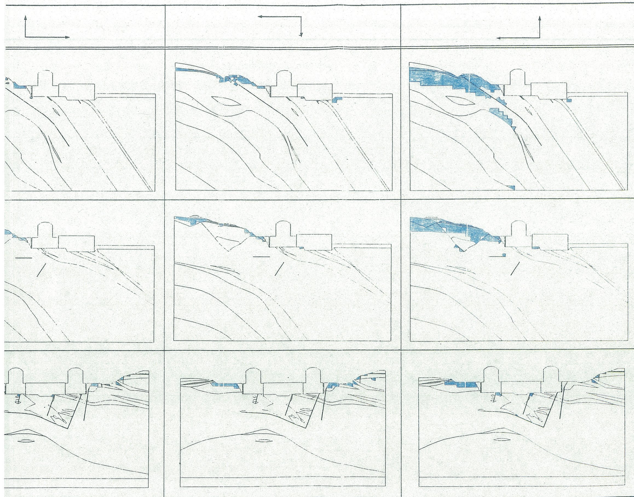
第 3.29 圖 静的線形解析 地震時引張領域分布一覽
