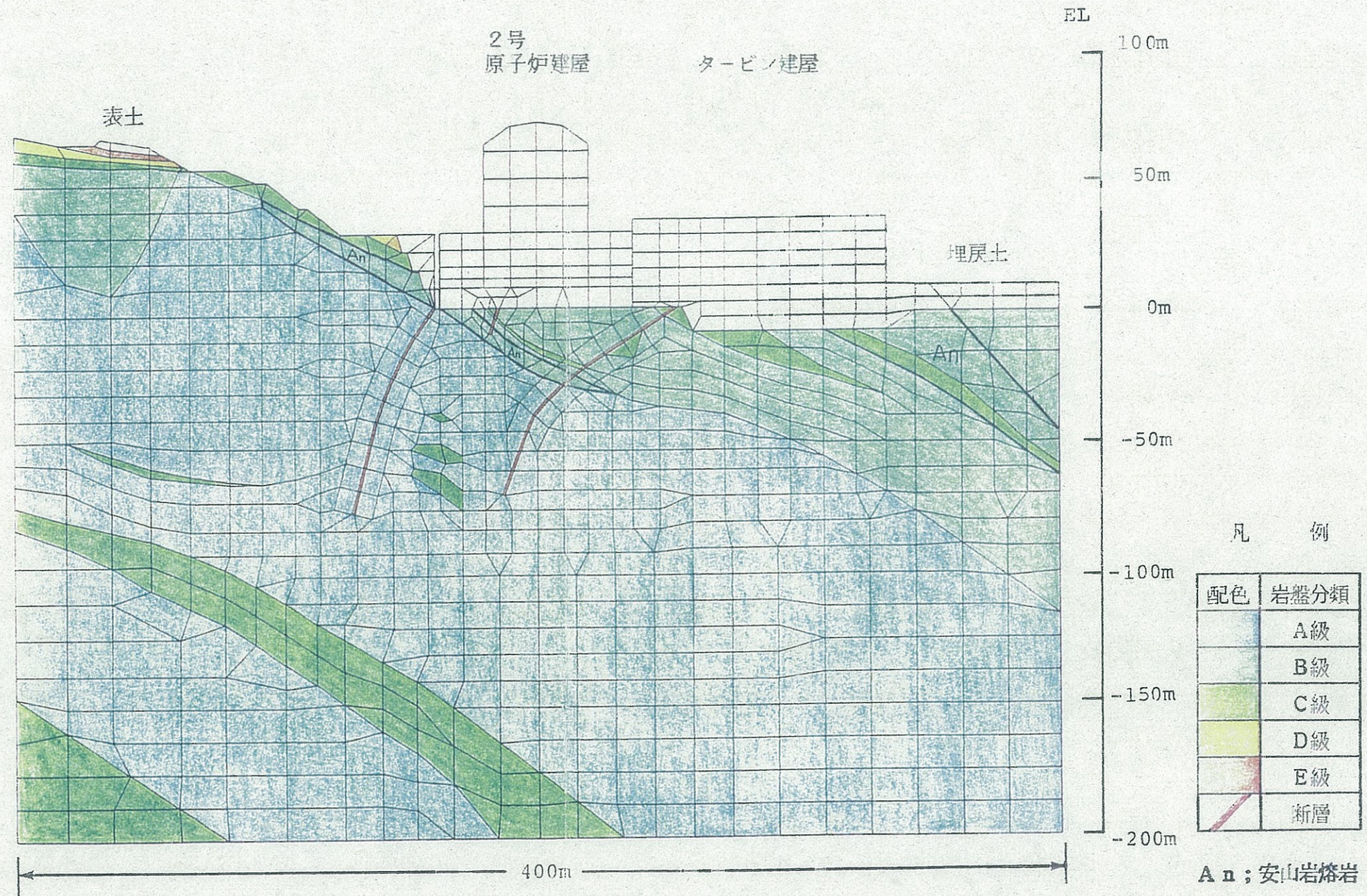
第2.21 図 静的FEM解析用要素分割図
