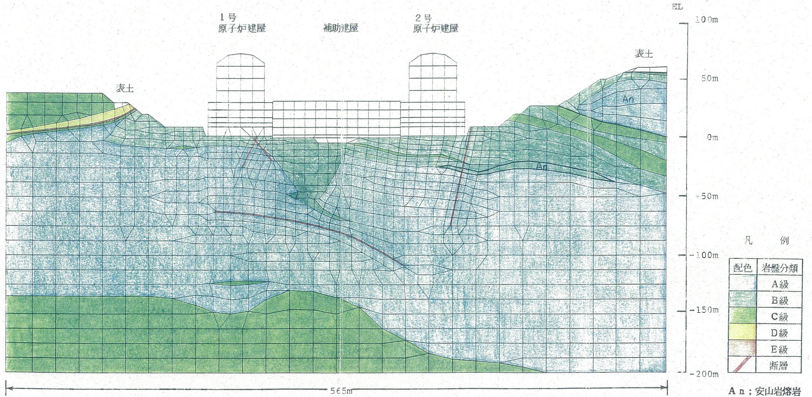
第2.22图 静的FEM解析用要素分割图
