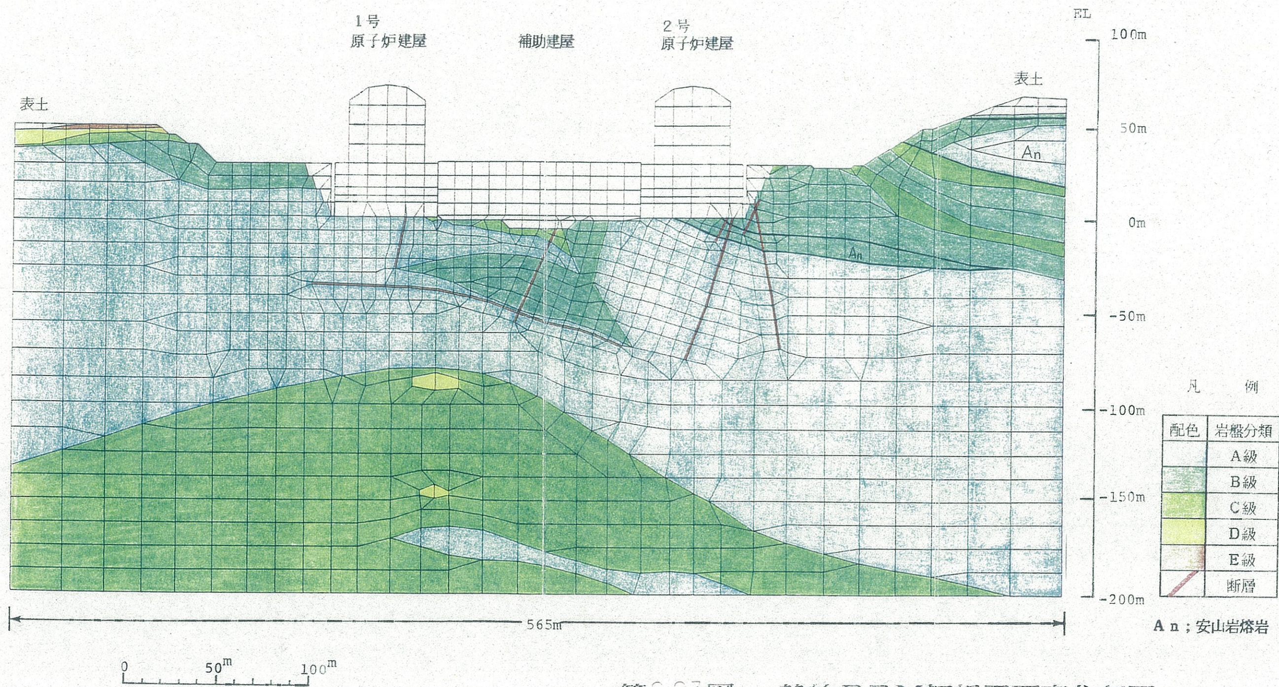
第2.23图 静的FEM解析用要素分割图
