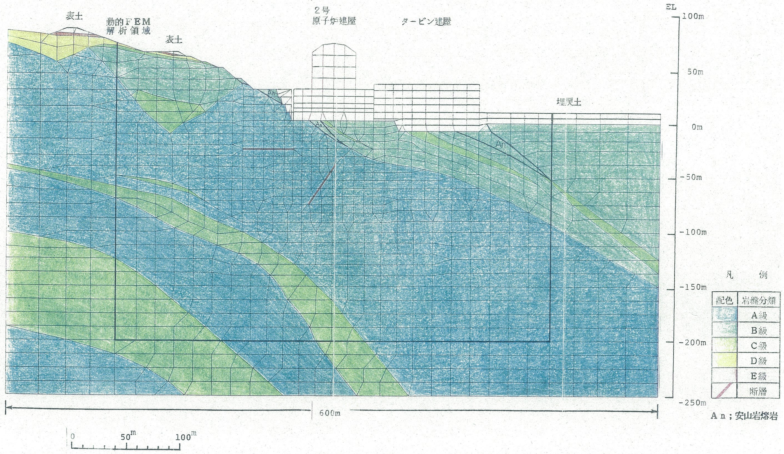
第2.16 図 動的FEM解析用要素分割図
