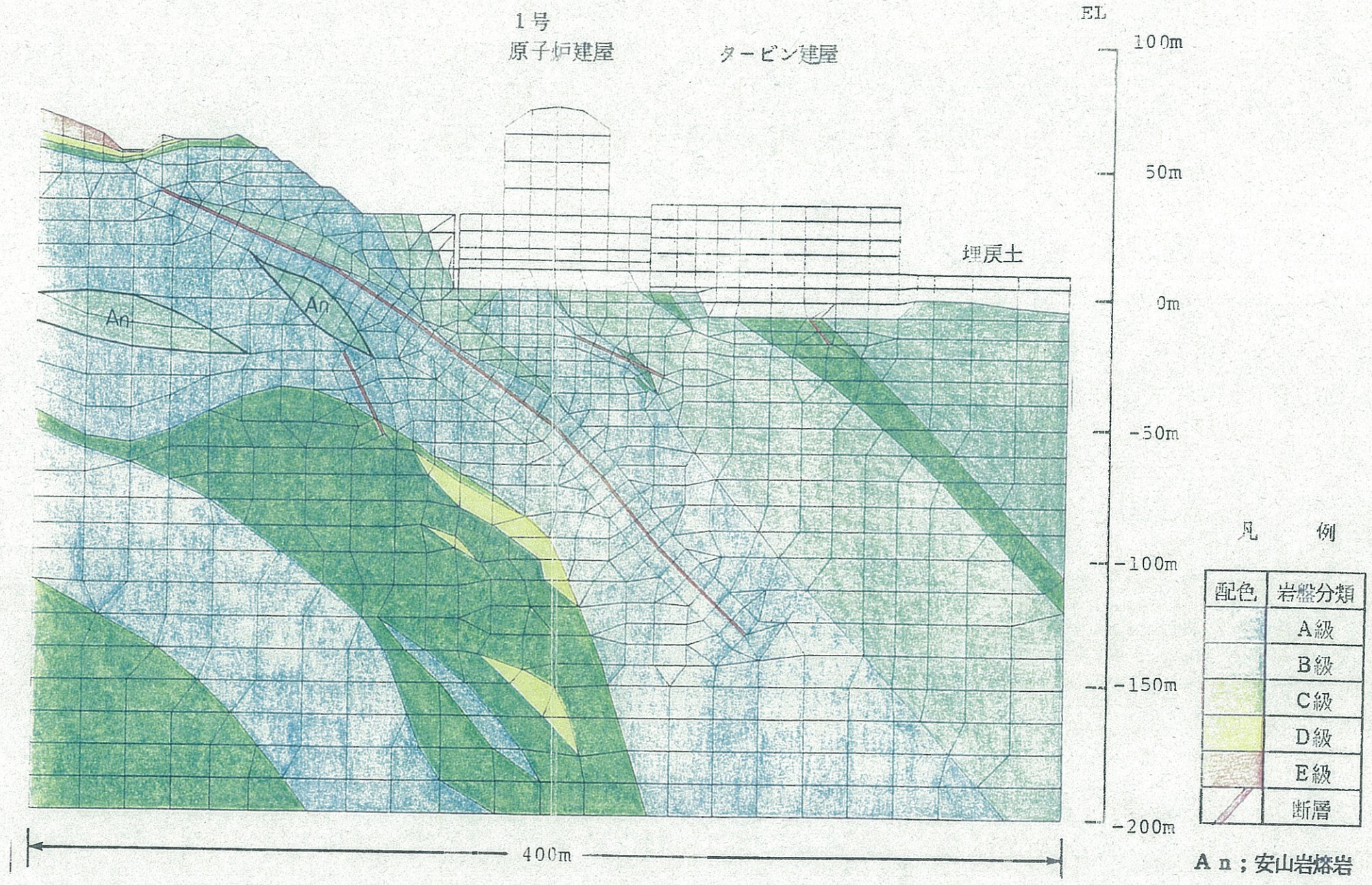
第2.19図 静的FEM解析用要素分割図
