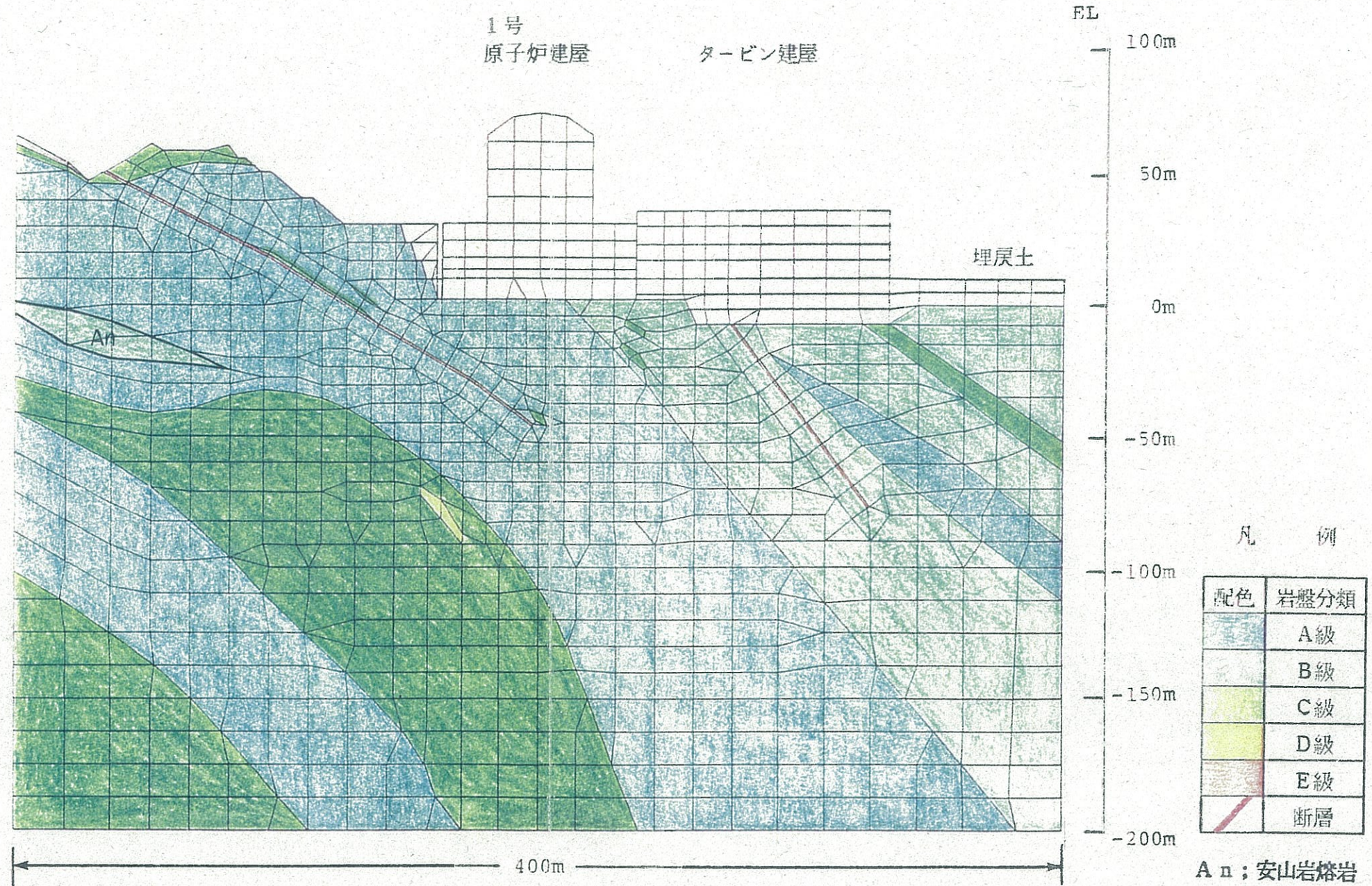
第 2.16 図 静的 FEM 解析用要素分割図
