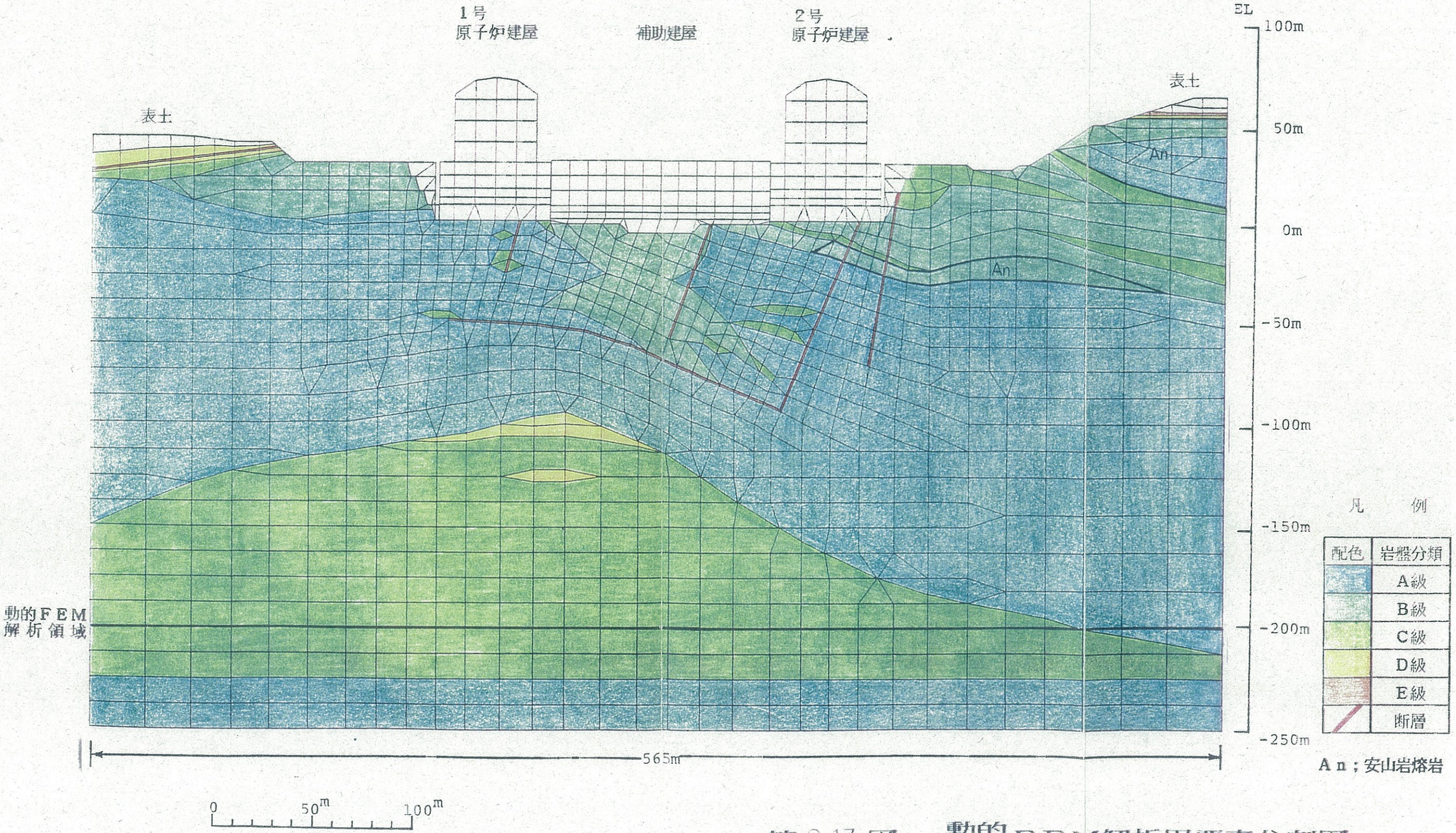
第 2.17 图 動的 FEM 解析用要素分割图
