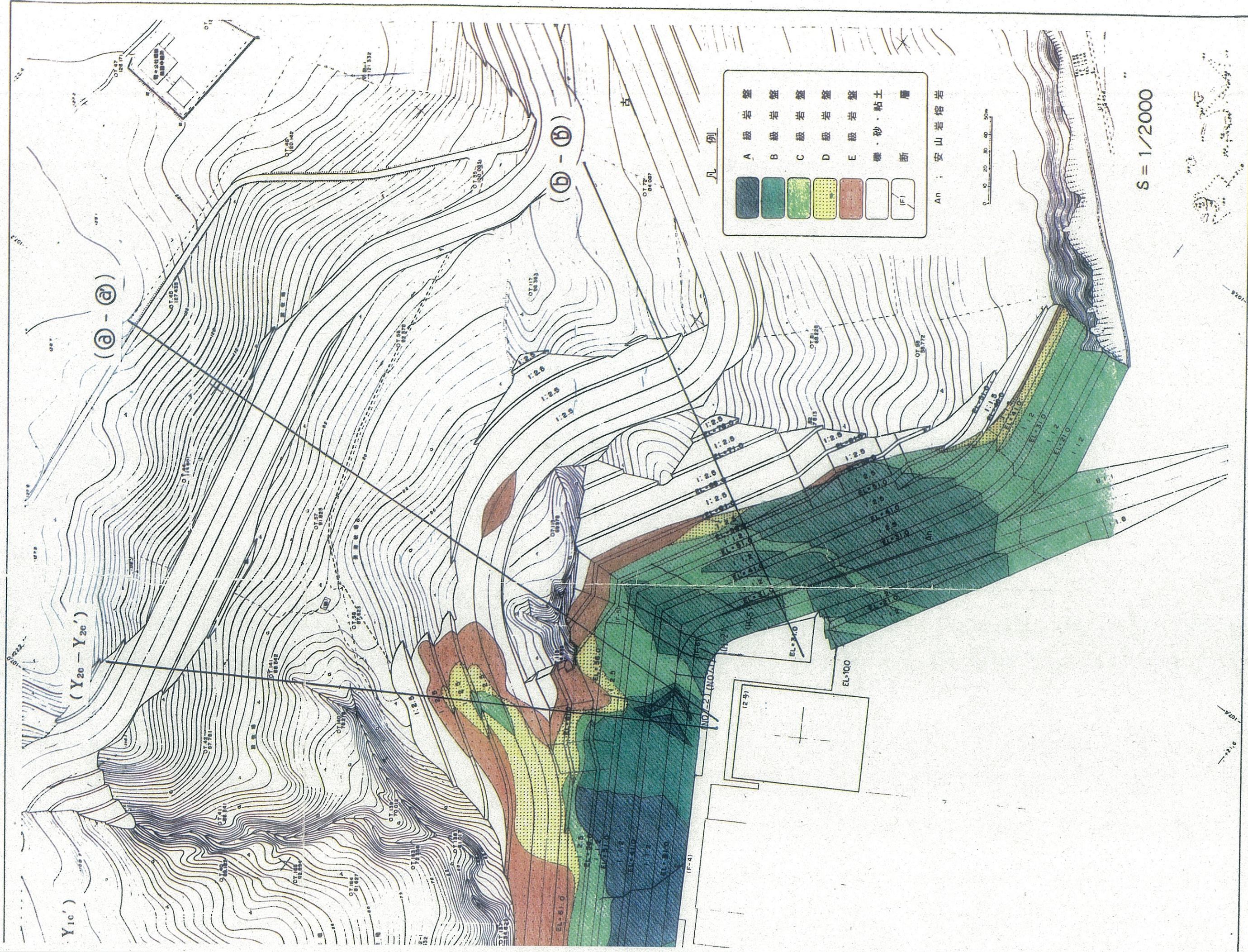
第 4.2.6 圖 水平岩盤分類圖
