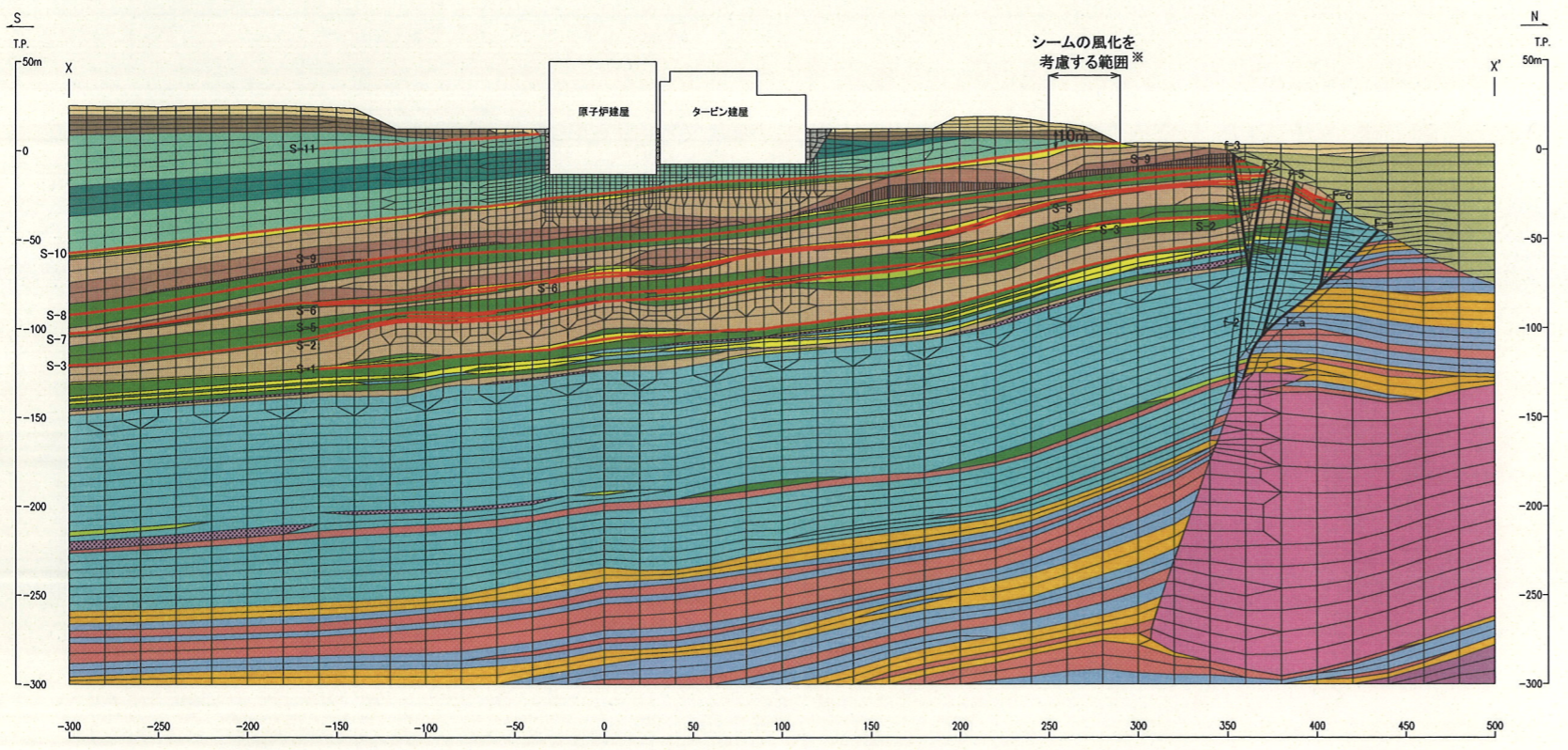
図-12 解析用要素分割図 (シームの風化部を考慮して強度特性を低減させた解析, X-X' 断面)
