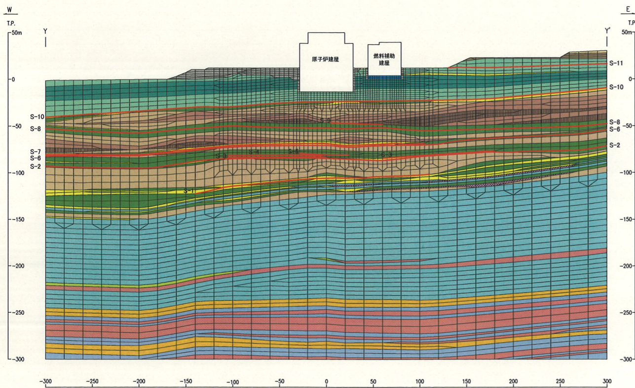
図-13 解析用要素分割図 (燃料補助建屋を付加したモデルによる解析, Y-Y' 断面)
