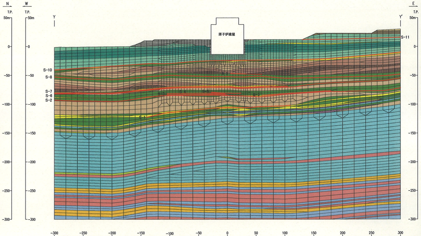
図-3(2) 解析用要素分割図(Y-Y'断面)
