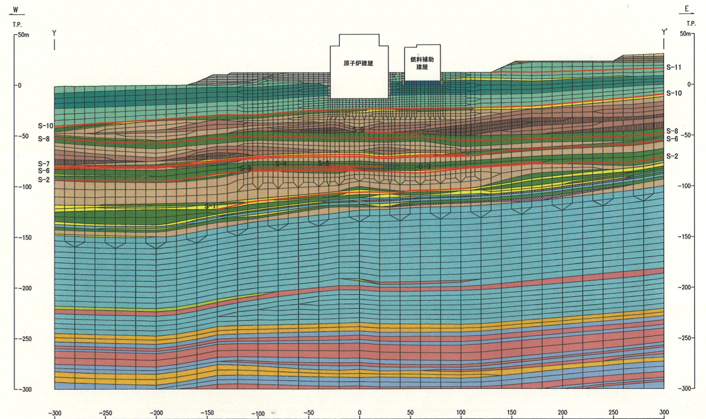
図-16(2) 解析用要素分割図(燃料補助建屋, Y-Y'断面)
