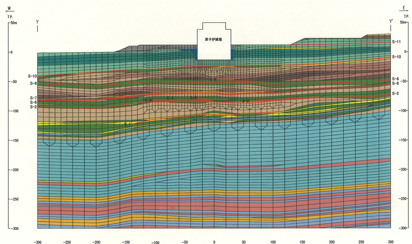
図-14(2) 解析用要素分割図 (T. P. +4.8mまでMMRによる建屋埋込み効果を考慮した解析, Y-Y' 断面)
