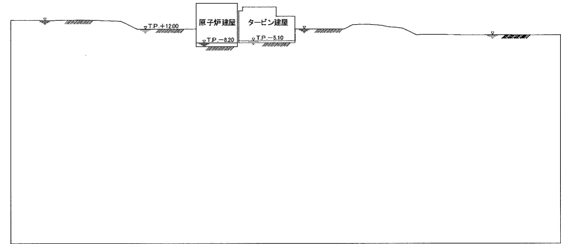
図-7(1) 地下水位設定図 (X-X' 断面)
