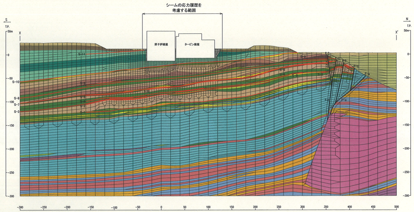
図-11 解析用要素分割図 (シームの応力履歴を考慮して強度特性を低減させた解析, X-X' 断面)
