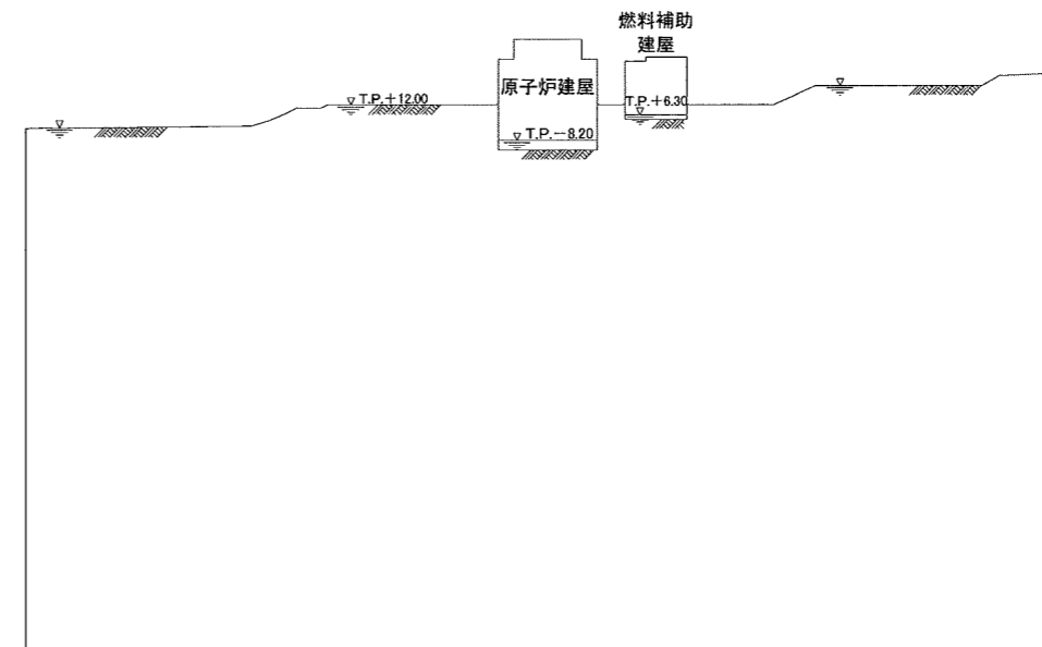
図-18(2) 地下水位設定図（燃料補助建屋，Y-Y' 断面）
