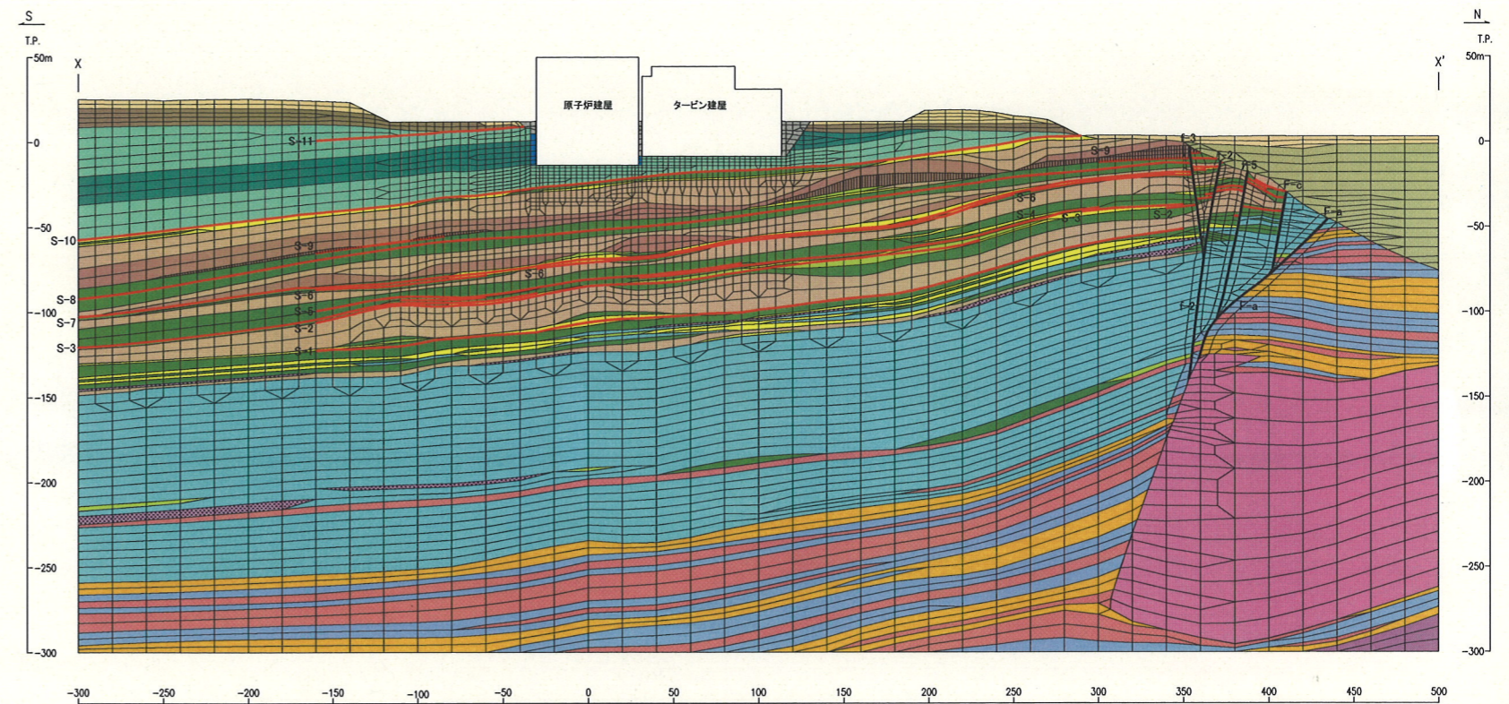
図-14(1) 解析用要素分割図 (T. P. +4.8mまでMMRによる建屋埋込み効果を考慮した解析, X-X' 断面)
