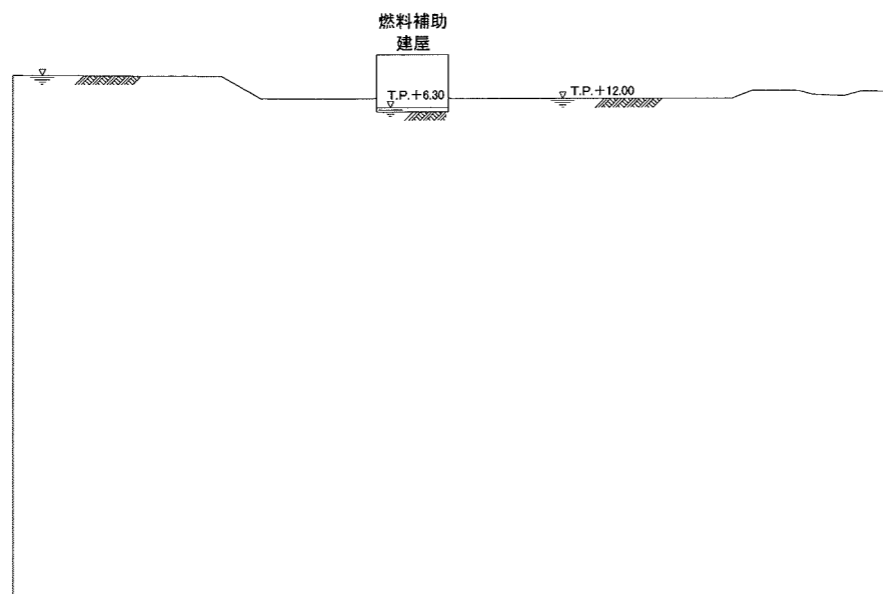
図-18(1) 地下水位設定図（燃料補助建屋，X-X' 断面）
