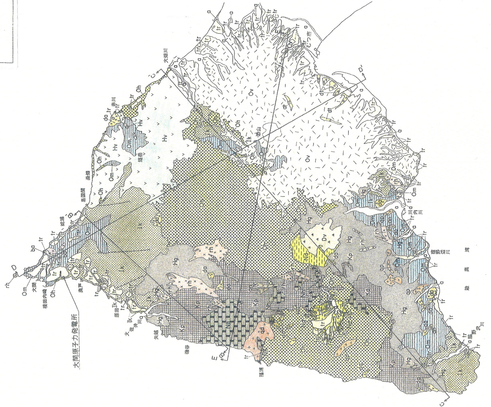
図-2 敷地周辺陸域の地質図
