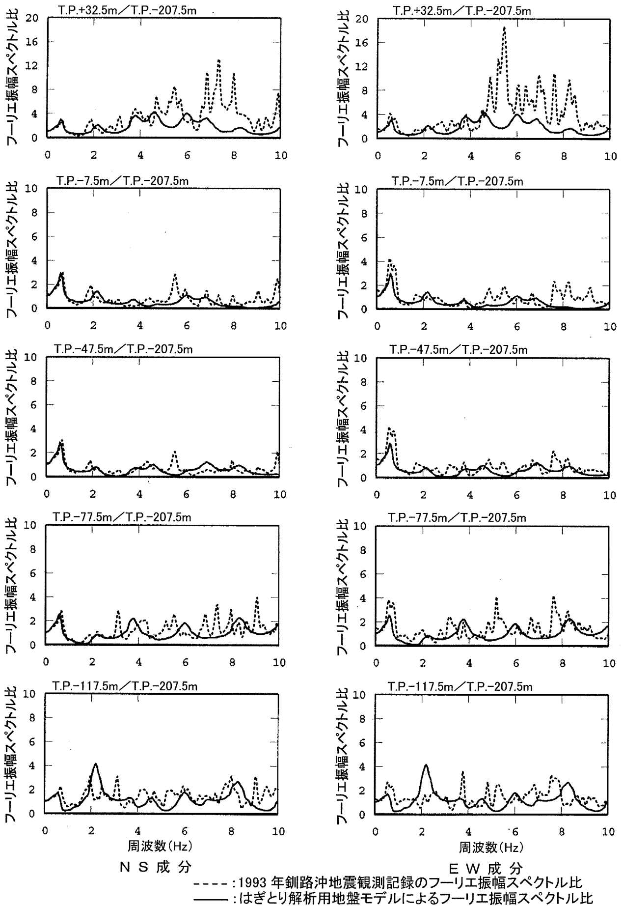
図-1.4 1993 年釧路沖地震観測記録とはぎとり解析用地盤モデルのフーリエ振幅スペクトル比の比較
