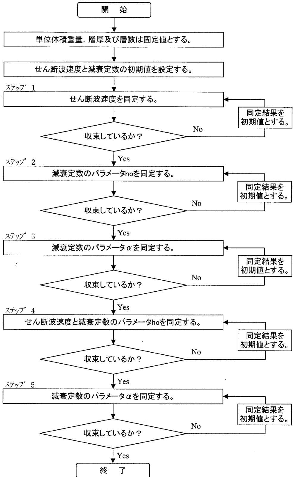
図-1.2 せん断波速度及び減衰定数の同定解析手順
