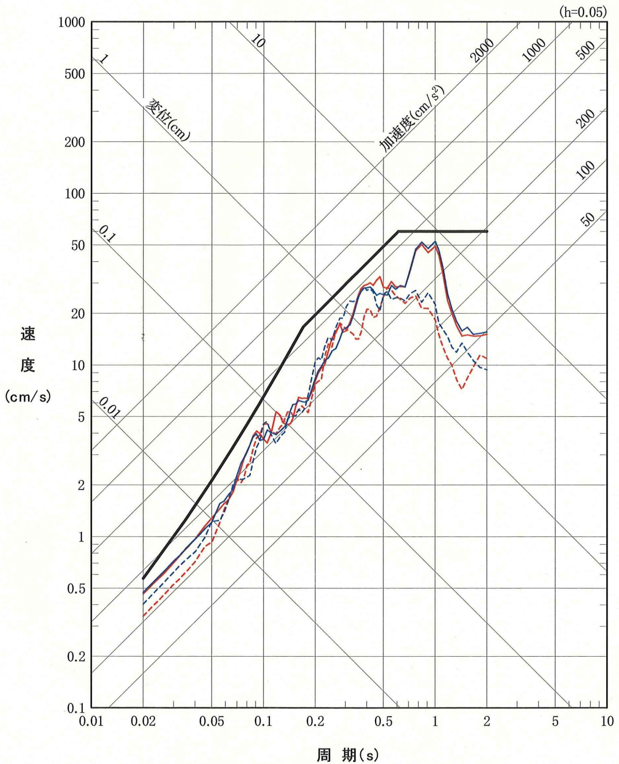
図-5 1993年釧路沖地震観測記録のはざとり波の応答スペクトルと設計用応答スペクトル S_1-D との比較(解放基盤相当位置) (はざとり解析用地盤の減衰定数は各層毎に設定)
