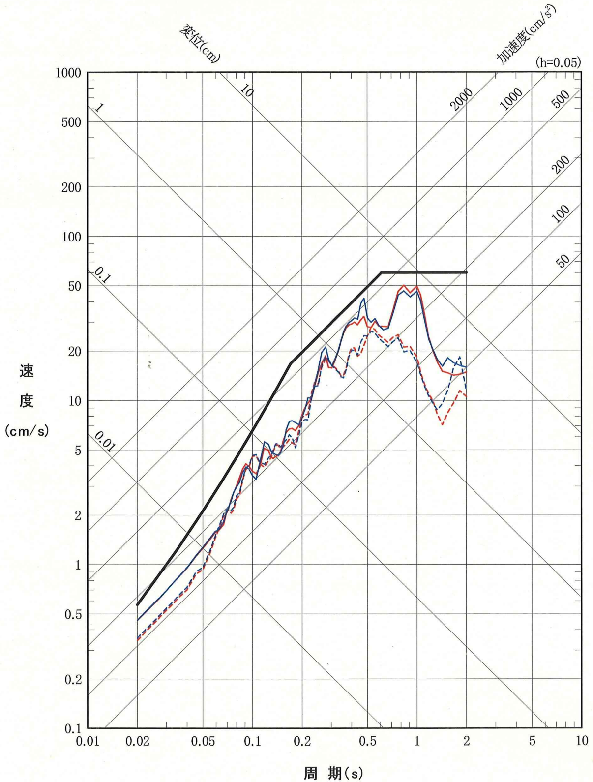
図-1.6 1993年釧路沖地震のはざとり波の応答スペクトル及び設計用応答スペクトル S_1-D (解放基盤相当位置)
