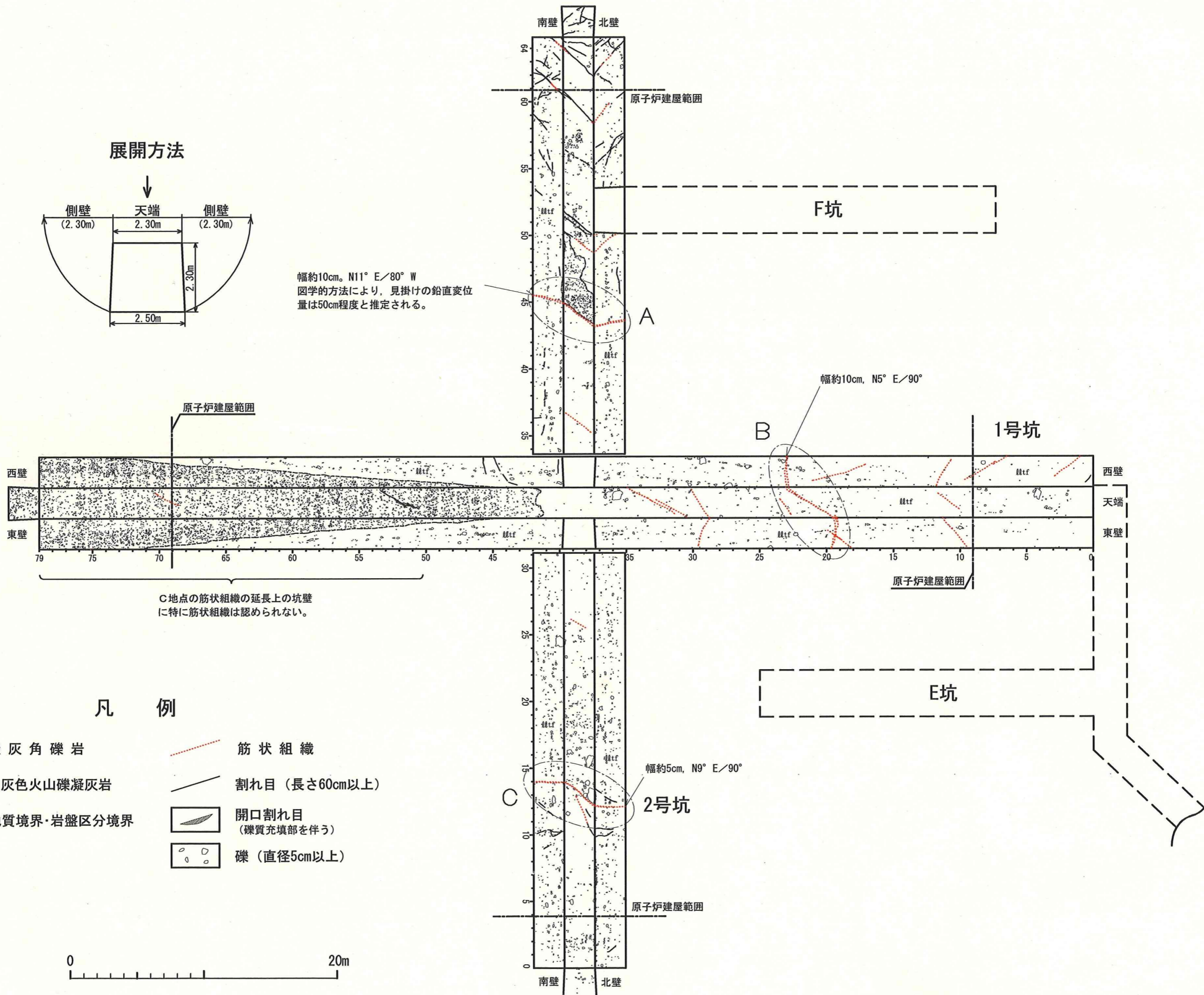
図-3.1 試掘坑における筋状組織の分布 3-2
