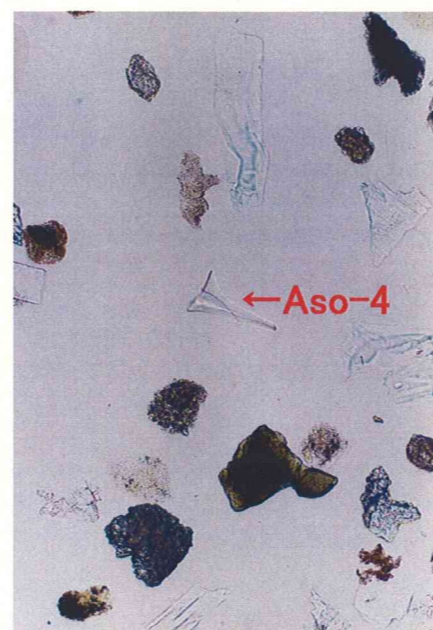
Ts-3 EE-18測線 深度(斜面上)0.45m
