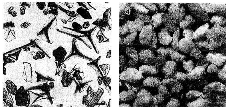
写真2 火山ガラスの形態を示す顕微鏡写真。 1. バブル型(平板状) …始良Tn火山灰(AT) 2. バブル型(Y字状) …阿蘇4火山灰(Aso-4) 3. 軽石型(繊維状) …鬼界幸屋(竹島)テフラ(K-Ky) 4. 軽石型(スポンジ状) …鬱陵隠岐火山灰(U-Ok) 5. 急冷破砕型(塊状) …立川ローム上部ガラス質火山灰(UG) スケール:1-3, 5は0.1mm; 4は1mm.
