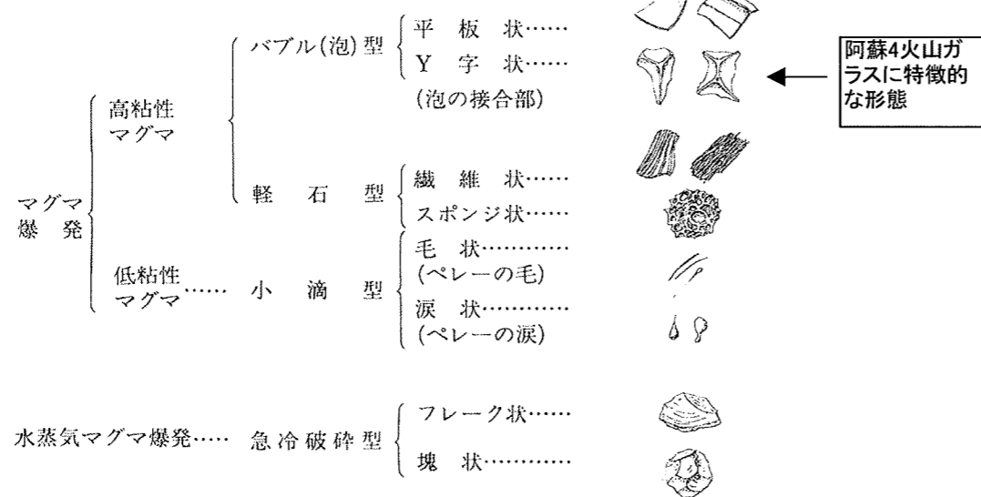
図6 火山ガラスの形態分類.
