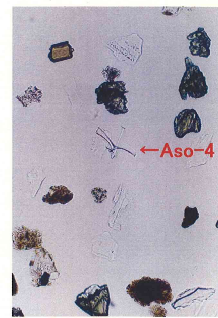
Ts-3 EE-36測線 深度(斜面上)0.85m
