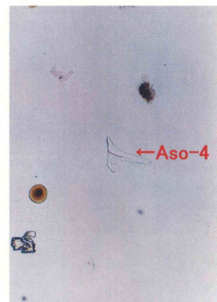
Ts-3 EW-36.5測線 深度(斜面上)0.65m
