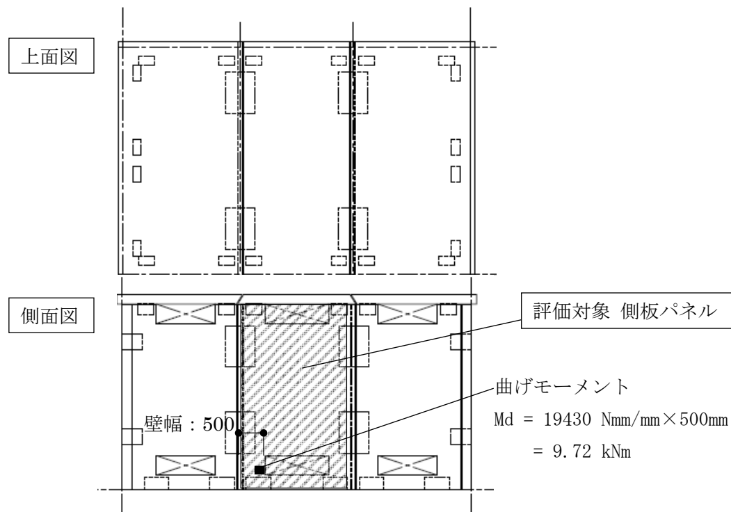
図 2.3-18 側板パネル
