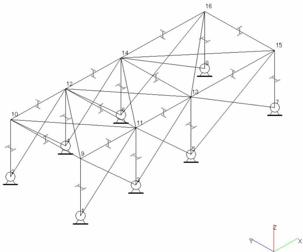
図－４ 凝集沈殿装置（アクチフロー）解析モデル
