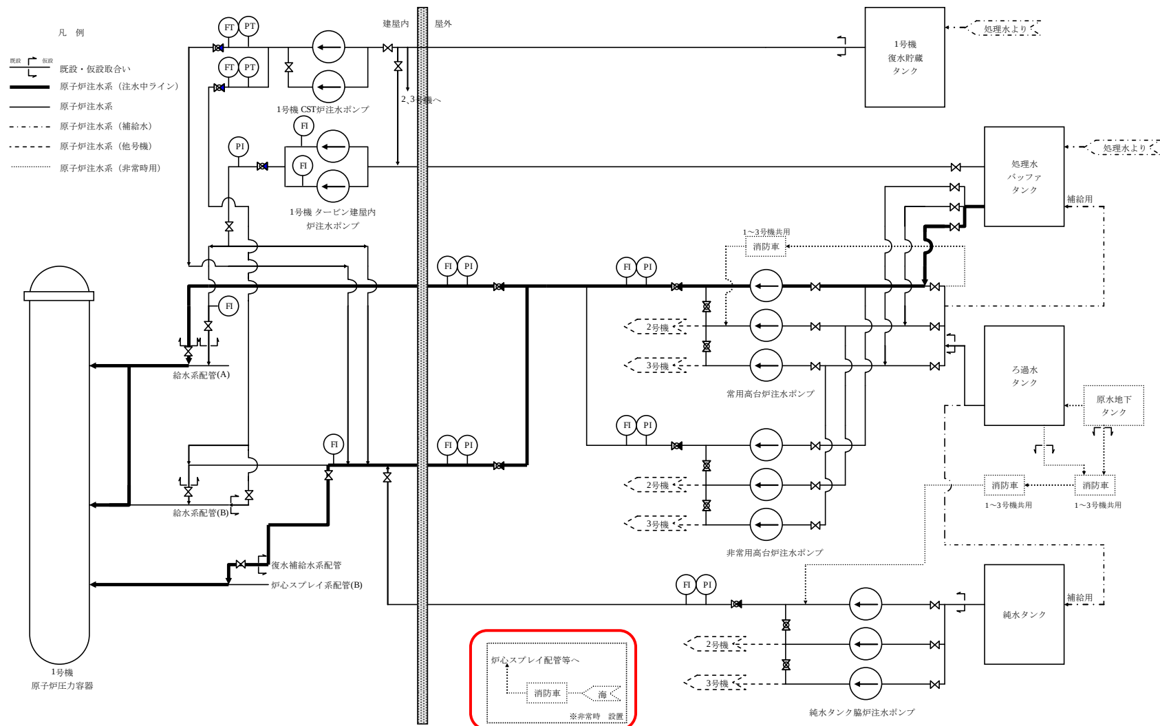
図ー 1 1号機原子炉压力容器・格納容器注水設備系統概略図
