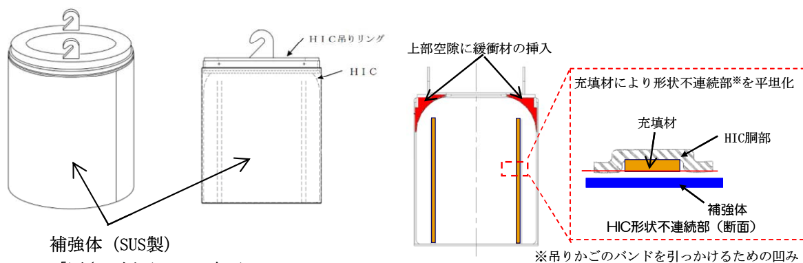
図 1 試験体
