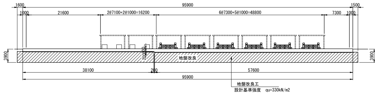
图 2.5-4 地盤改良断面図 (单位: mm)
