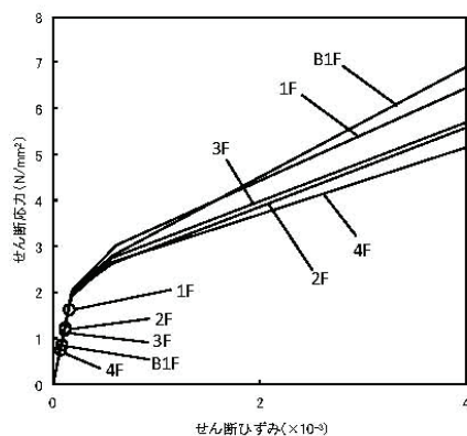
せん断スカルトン曲線上の最大応答値 (Ss-1、EW方向)
