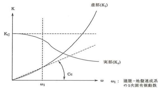
図-4.3 地盤ばねの近似
