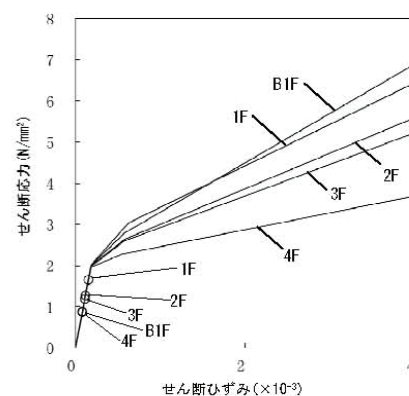
【参考】平成22年耐震バックチェック*時における せん断スカルトン曲線上の最大応答値 (Ss-1、EW方向)
