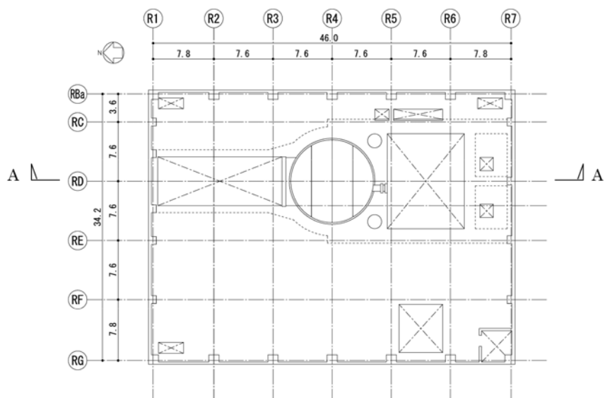
图-1.1 5 阶 (OP 39.92) 平面图 (单位 : m)
