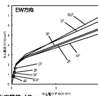
せん断スkeleton曲線上の最大応答値（Ss-1）
