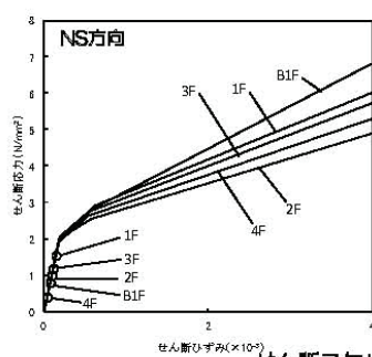
せん断スkeleton曲線上の最大応答値（Ss-1）
