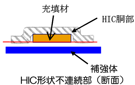
図2 HIC 補強概要
