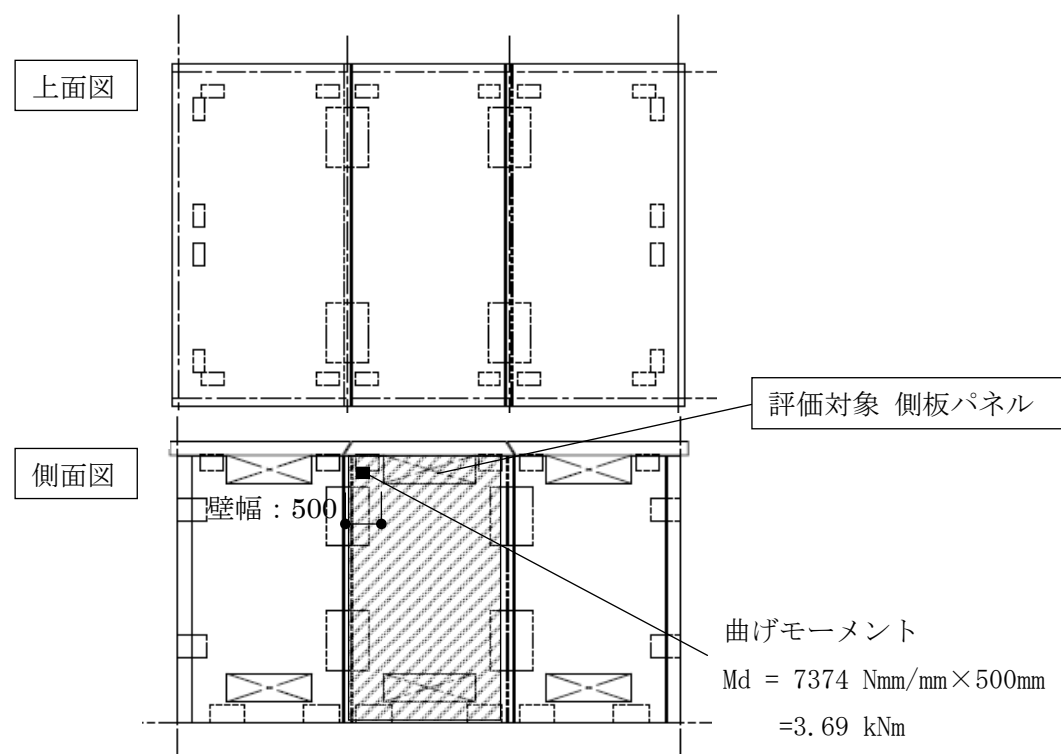
図 1.2-5 側板パネル
