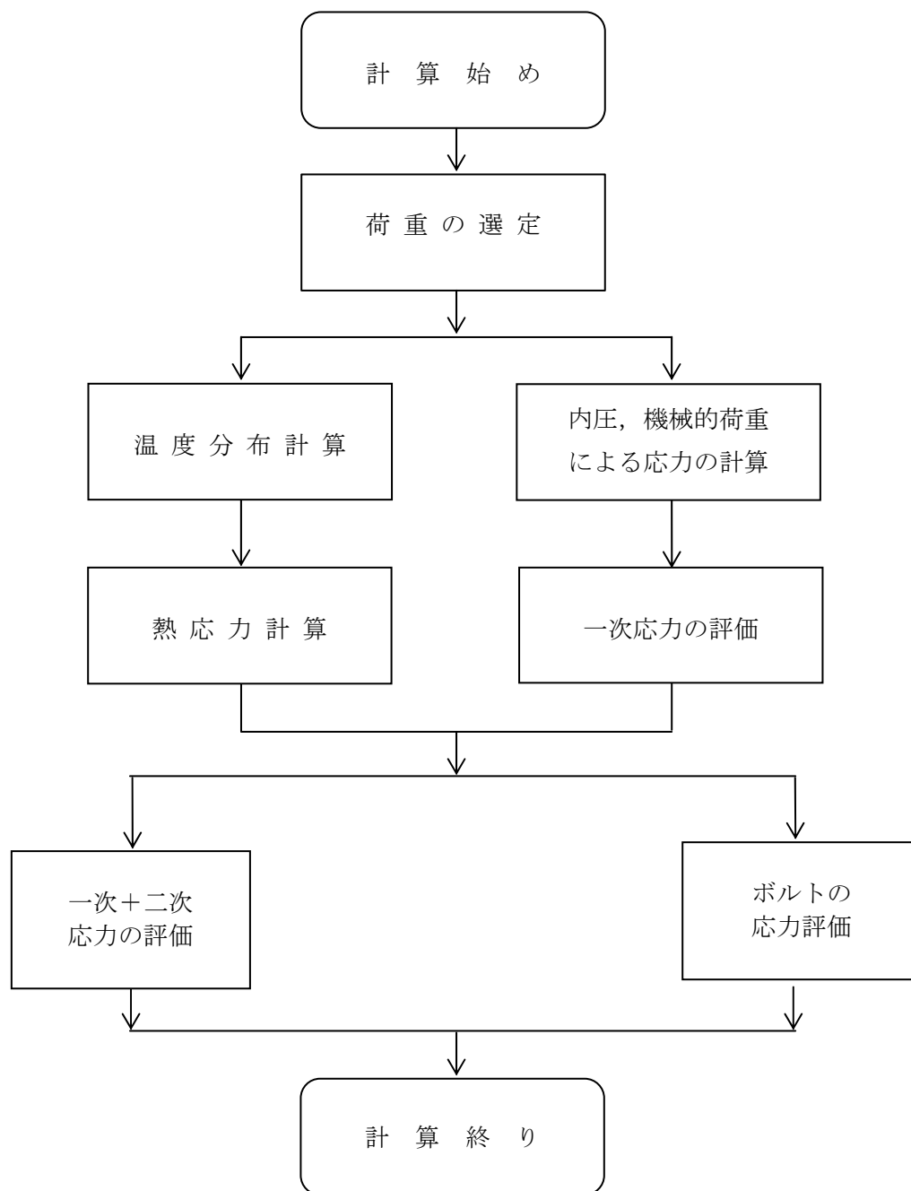
図 2.1-8 8 キャスク容器及び二次蓋の応力解析フロー図
