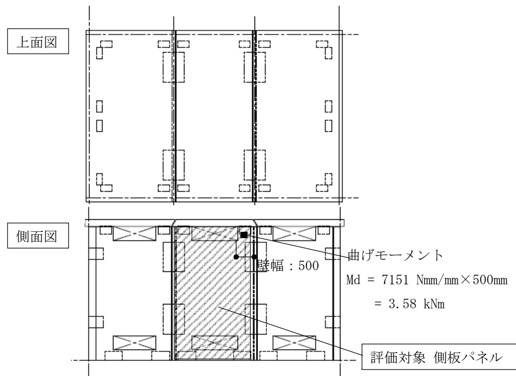
図 1.2-10 側板パネル
