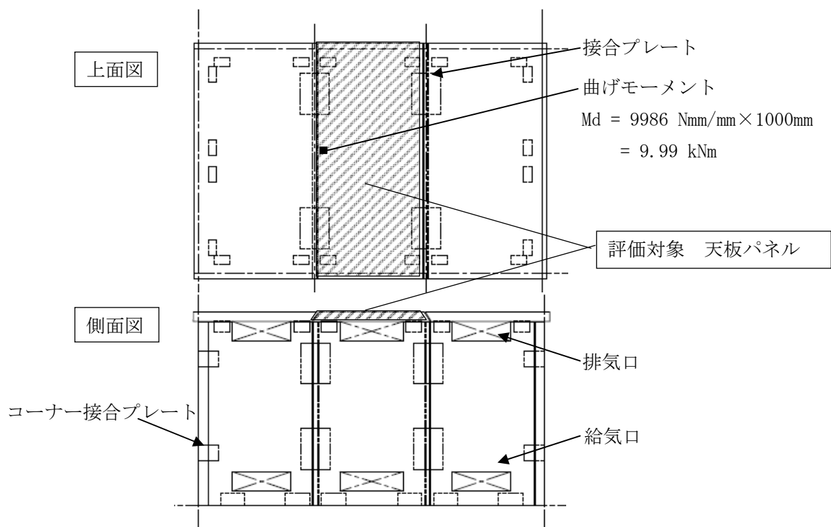
図 2.3-7 天板パネル
