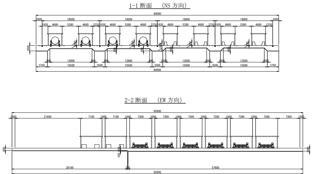
图 1.4-3 基础断面图 (单位: mm)
