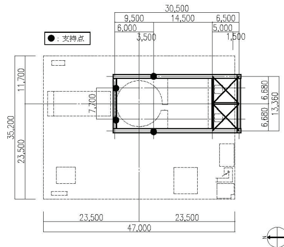
図-1.4.2 燃料取扱機支持用架構 梁伏図 (0.P. 41, 420)
