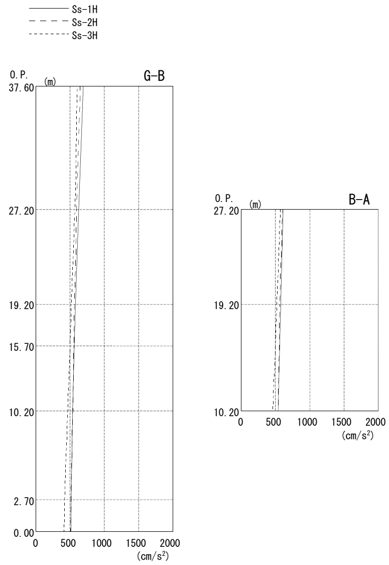
図9 PL/B 最大応答加速度(NS方向)
