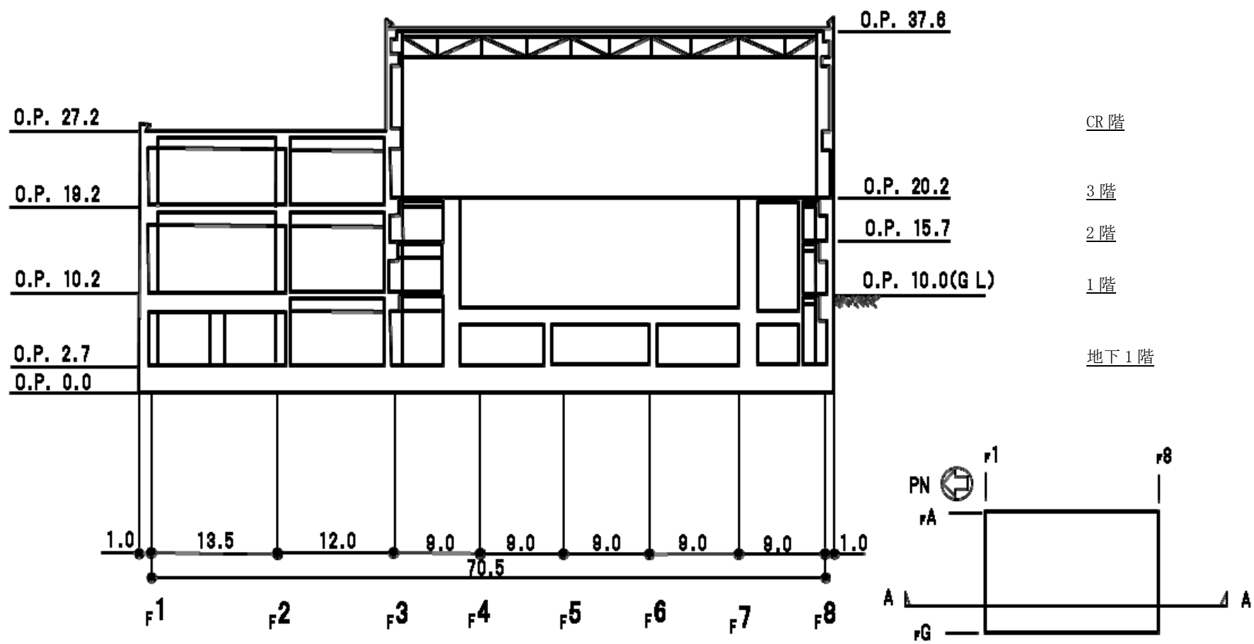
図2 PL/B NS方向断面図 (単位：m)
