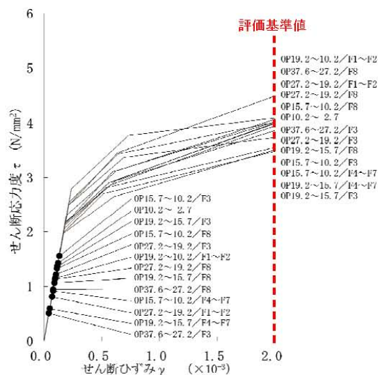
せん断スケルトン曲線上的最大応答値 ( S_s-2 EW方向)
