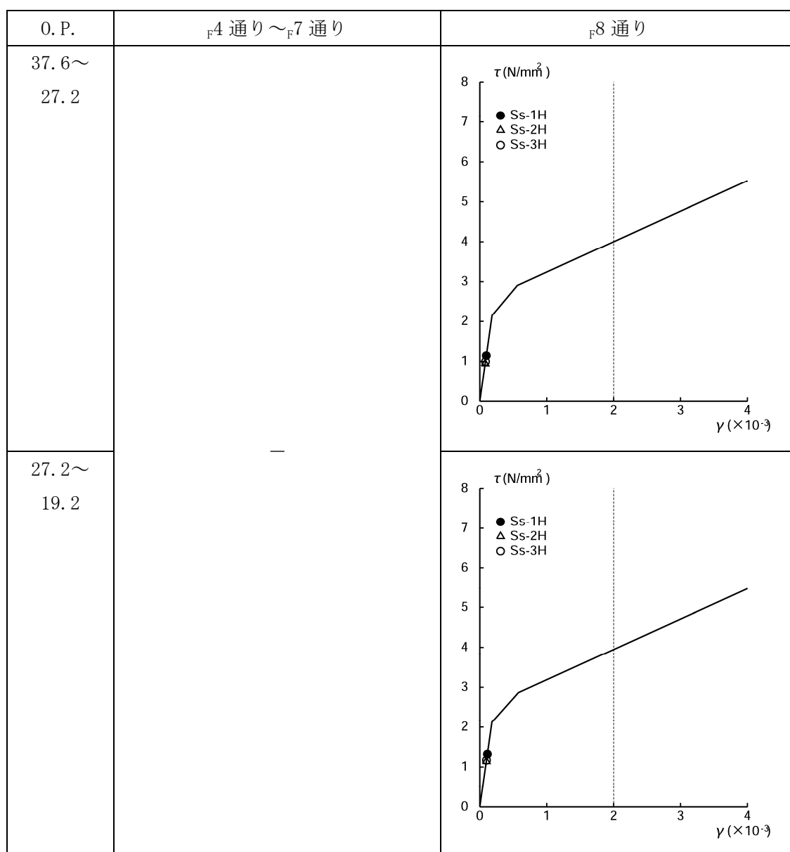
図 12 (3) PL/B せん断スケルトン曲線上の最大応答値 EW 方向
