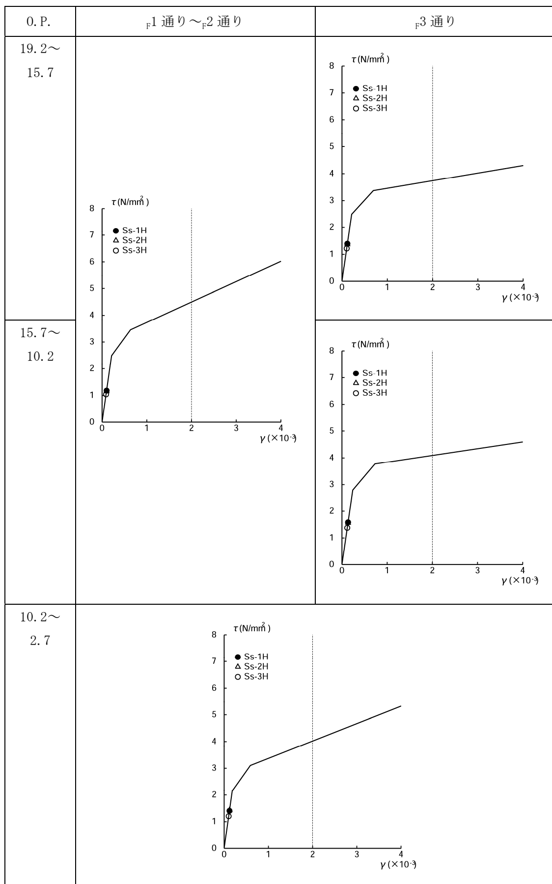
図 12(2) PL/B セン断スケルトン曲線上の最大応答値 EW 方向
