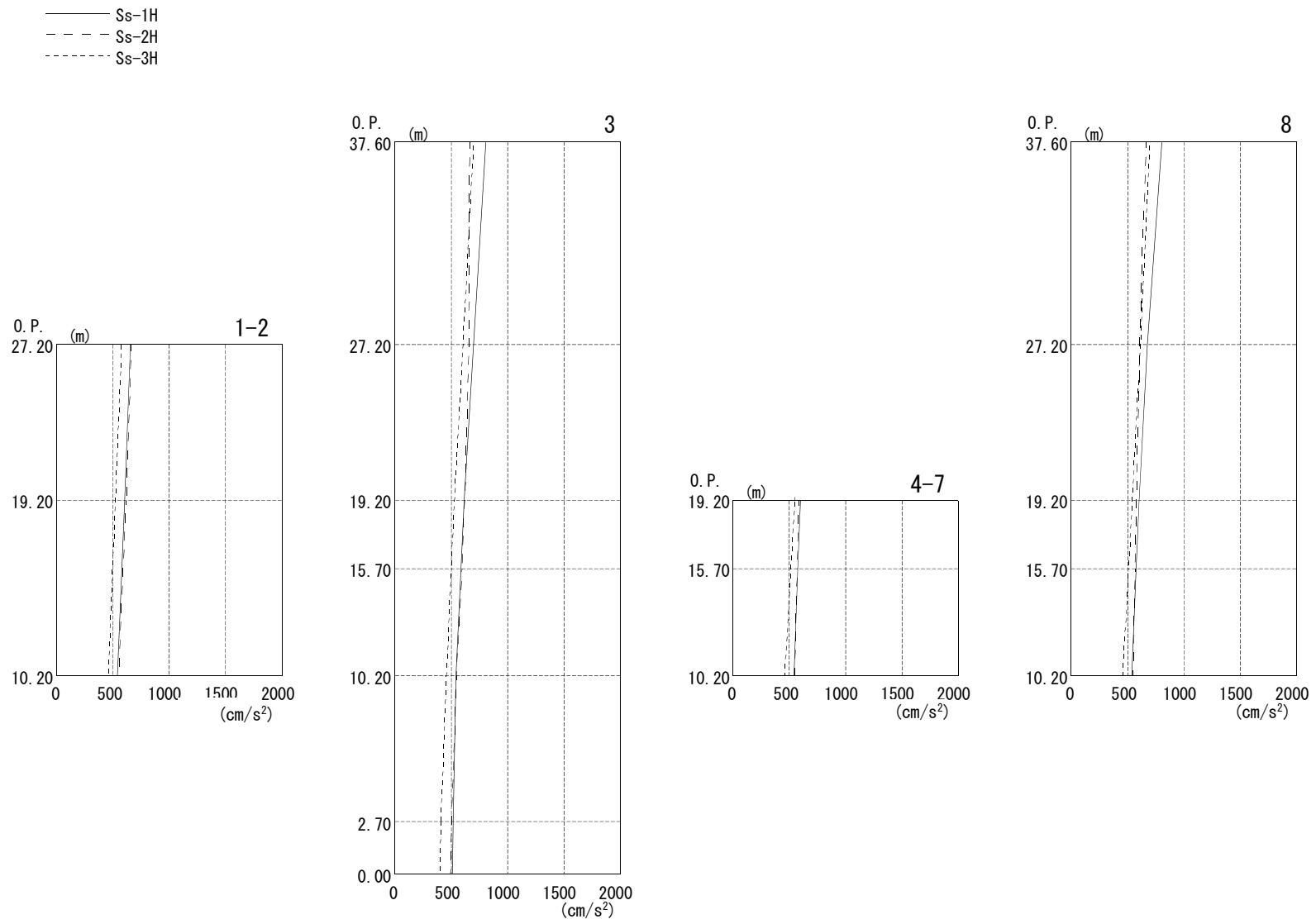
図10 PL/B 最大応答加速度(EW方向)
