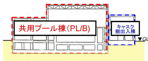
共用プール棟 (PL/B) ・ガスク搬出入棟 NS方向断面図
