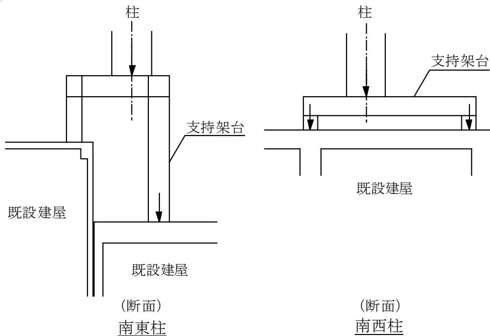
図 2-4 支持架台
