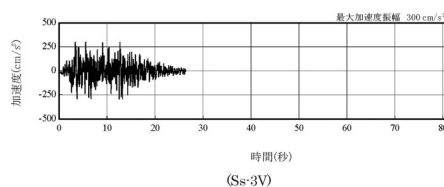
解放基盤表面位置における地震動の 加速度時刻歴波形(鉛直方向)
