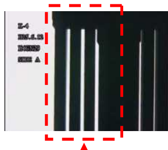
C面からの透過光による 燃料棒-ウォーター・ロッド間隔の A面からの確認
