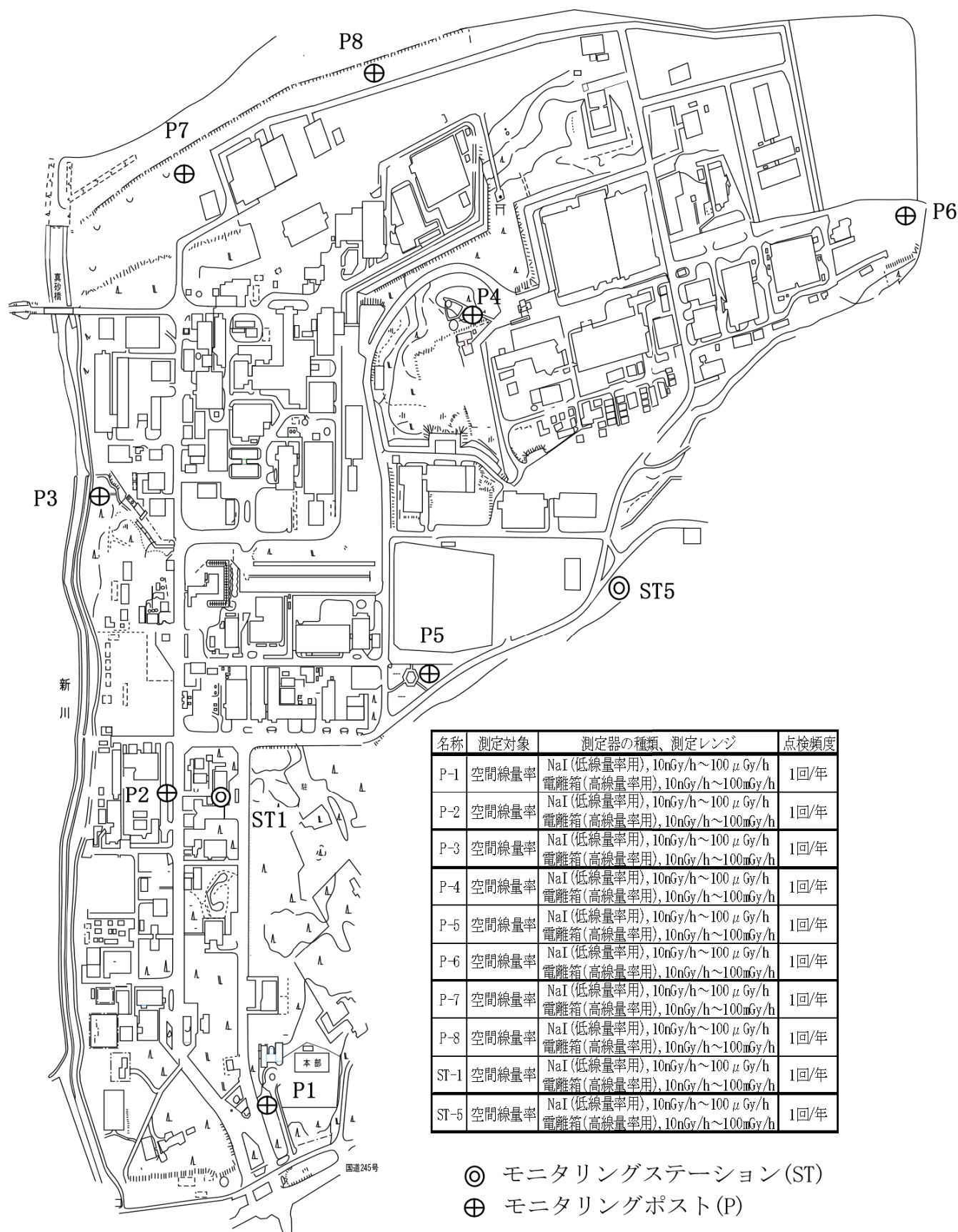
別図ー 4 サイクル研究所敷地周辺の放射線測定設備
