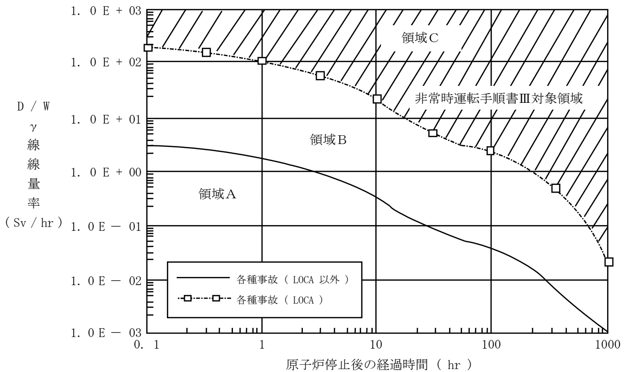
図3 ドライウェル領域の事故時放射線モニタ γ線線量率
