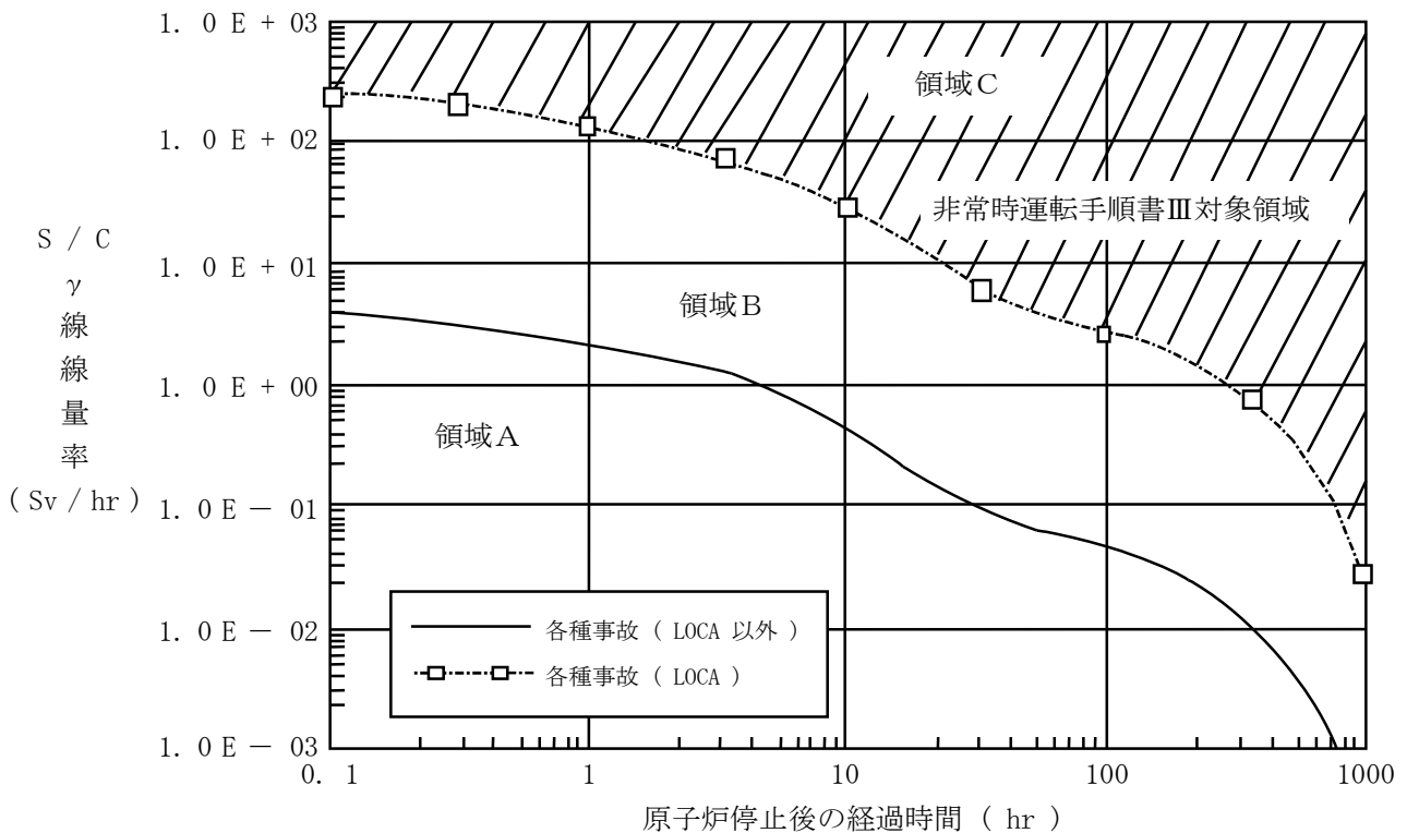
図4 サプレッション・チェンバ領域の事故時放射線モニタ γ線線量率
