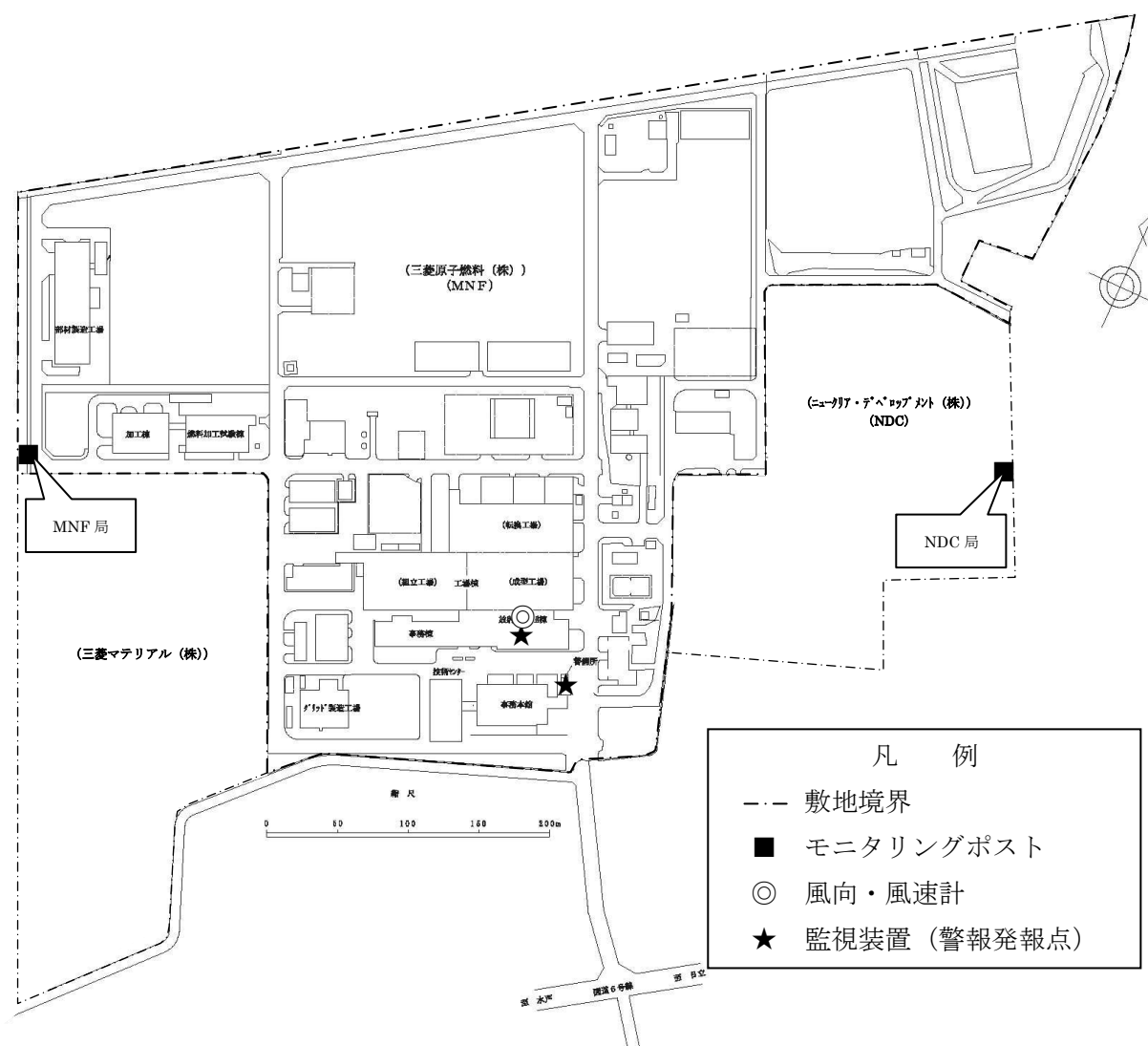
別図第6 「事業所敷地周辺の放射線測定設備及びその他の設備」
